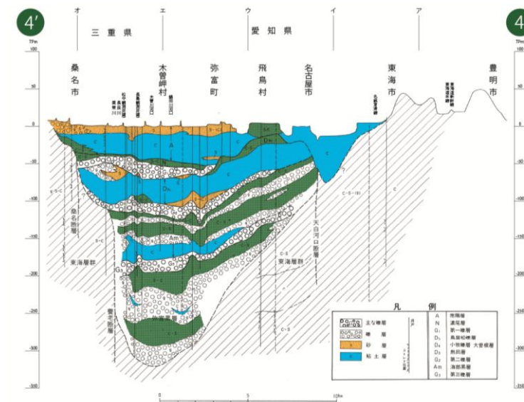
付図一4(4) 地層断面図④～④'
