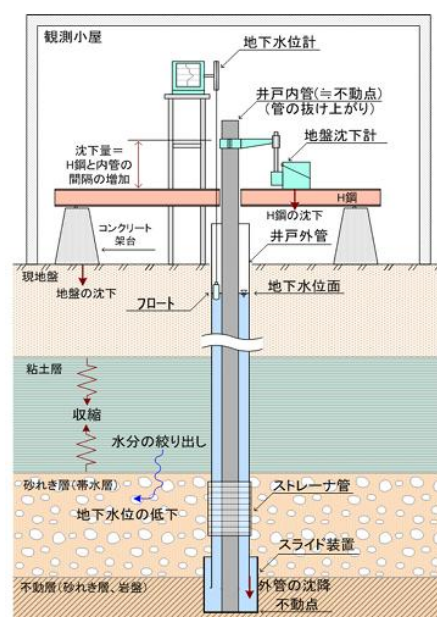
二重管式観測井の構造例
