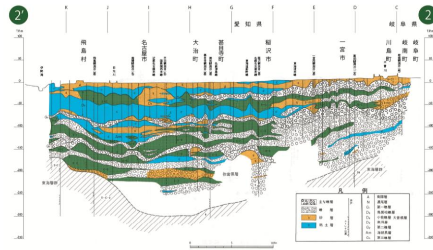
付図一4(2) 地層断面図②～②'
