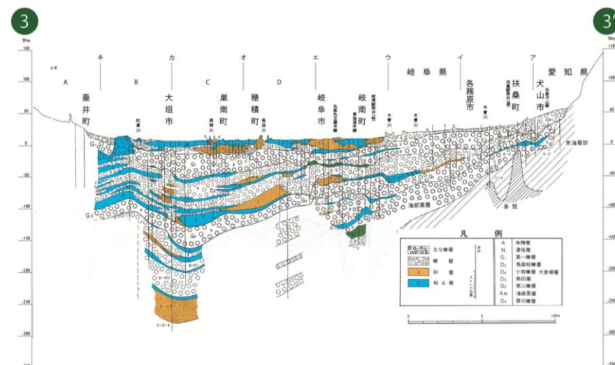
付図一4(3) 地層断面図③～③'
