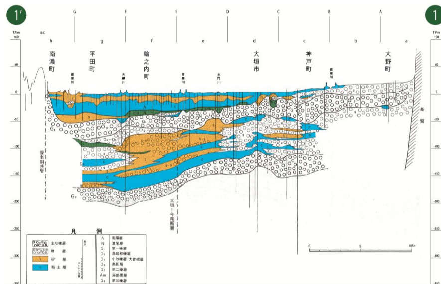
付図—4(1) 地層断面図①～①'
