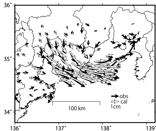
観測値(黒)と計算値(白)の比較 (2022-01-01/2026-06-18)
