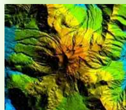
高精度地形データ
