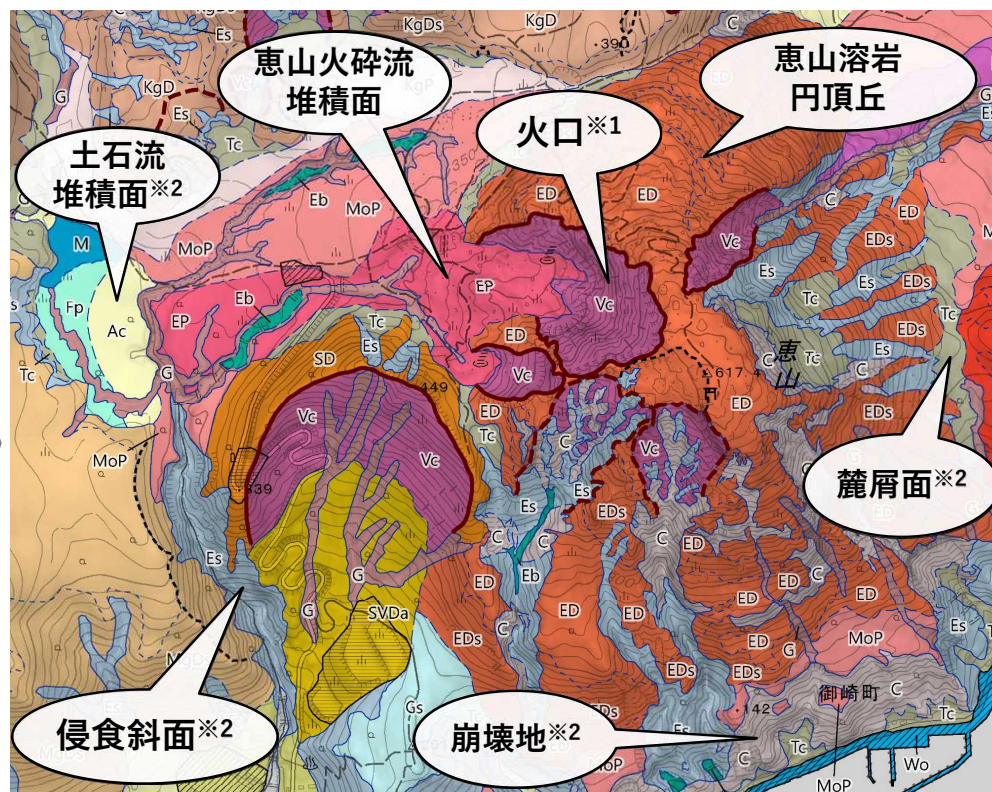
火山土地条件図「恵山」の一部
