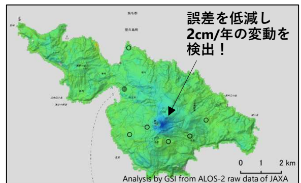
干渉SAR時系列解析結果
