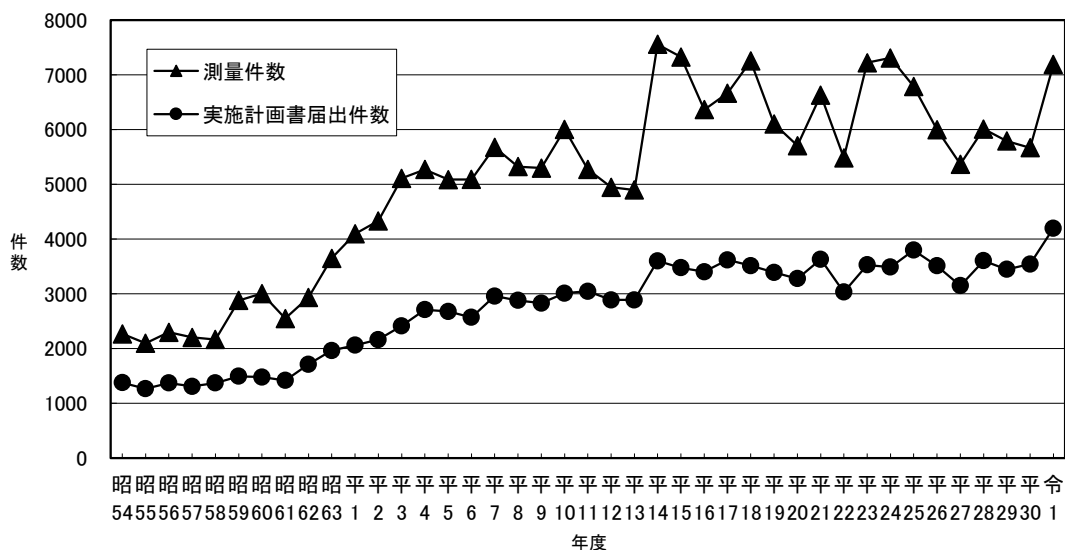
図-1 公共測量実施計画書届出件数と測量件数の推移 (昭和54年度～令和元年度)
