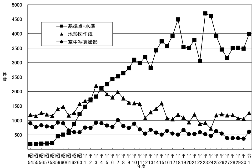
図-2 主な測量の測量件数の推移 (昭和54年度～令和元年度)
