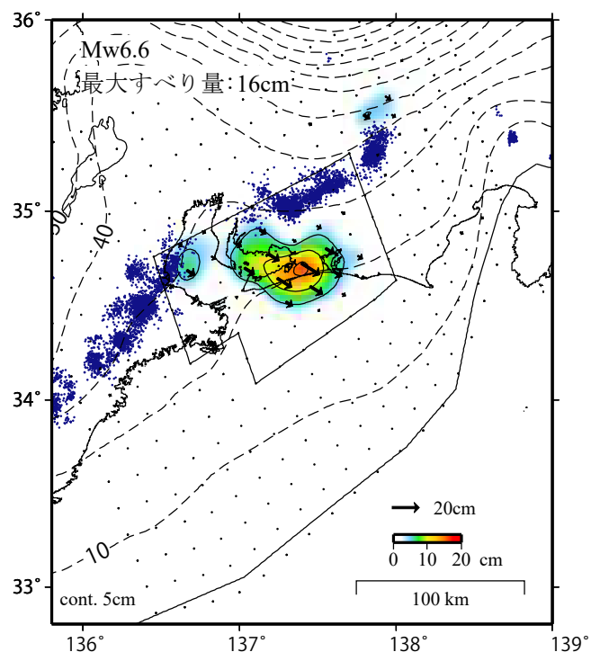
推定すべり分布 (2022-01-01/2025-08-22)
