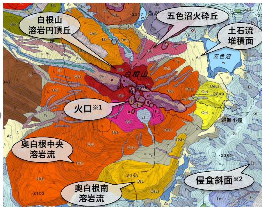
火山土地条件図「日光白根山」の一部
