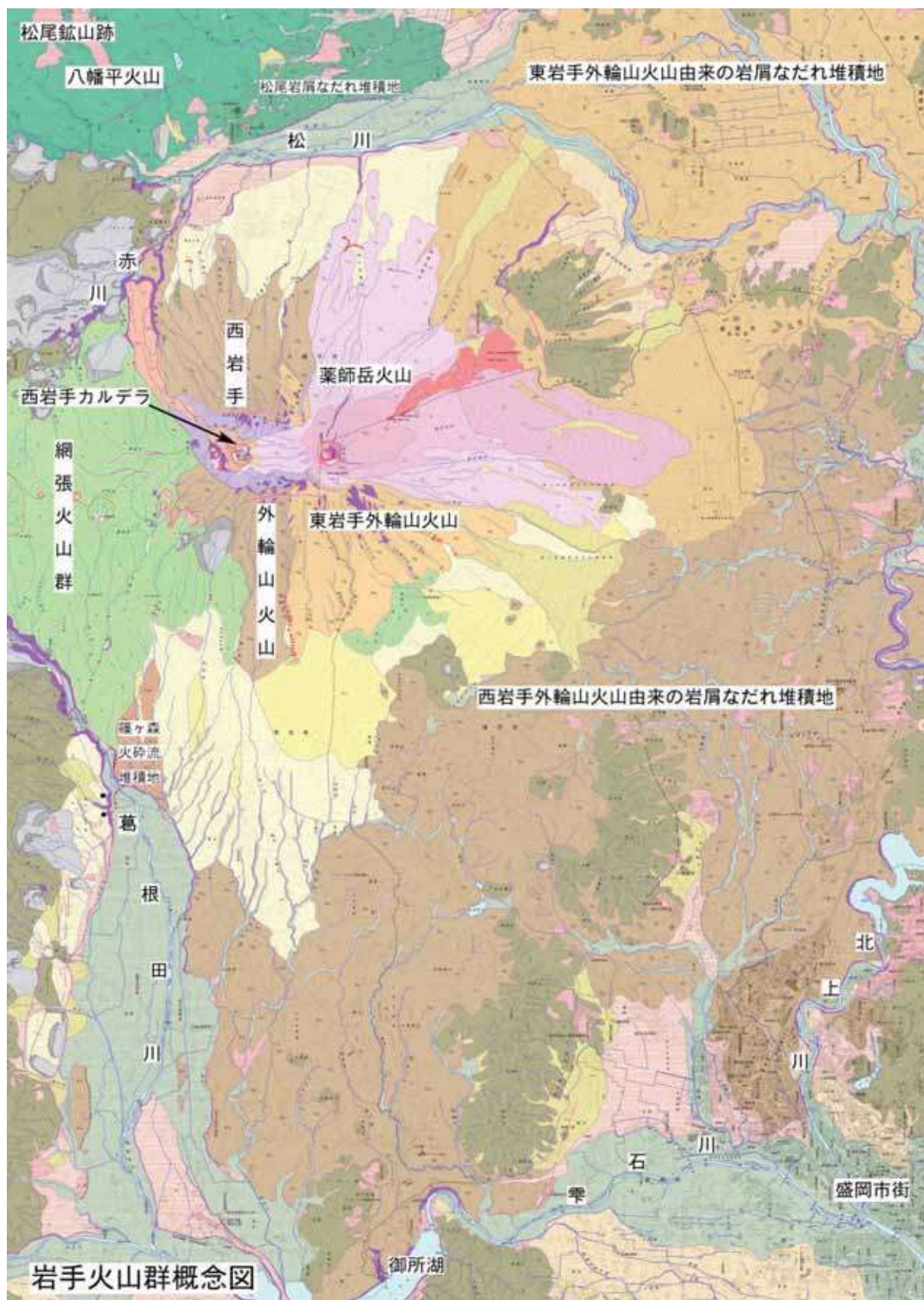
図－４ 岩手火山概念図
