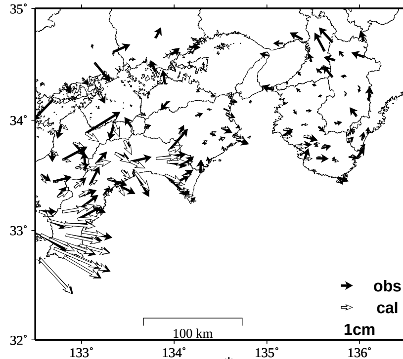
観測値（黒）と計算値（白）の比較 (2019-01-01/2024-06-11)
