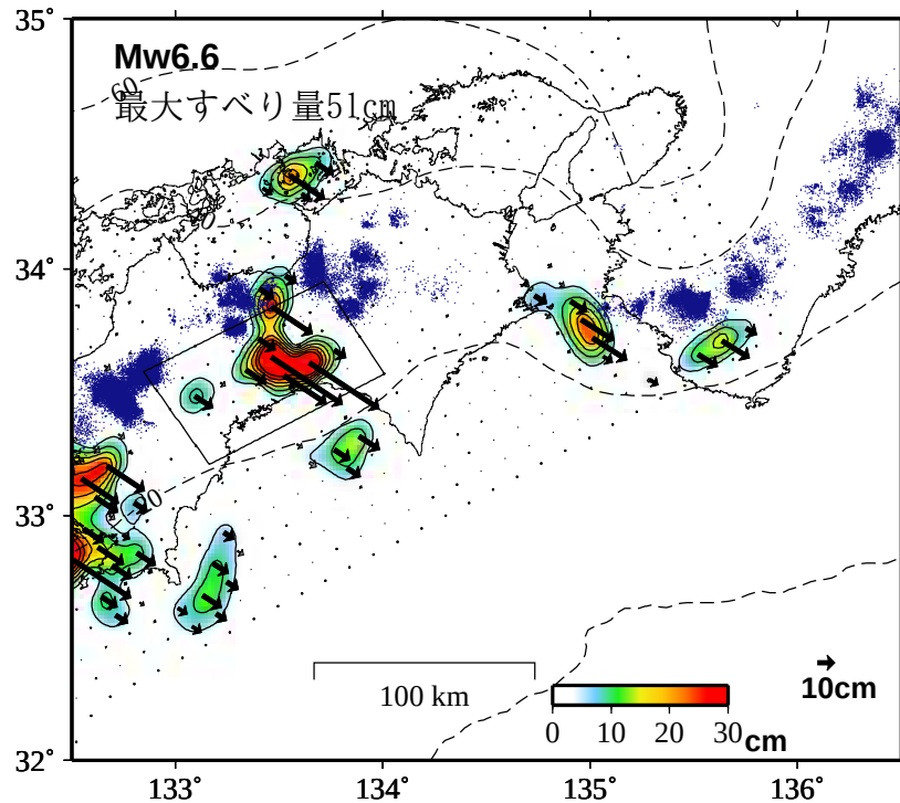
推定すべり分布 (2019-01-01/2024-06-11)
