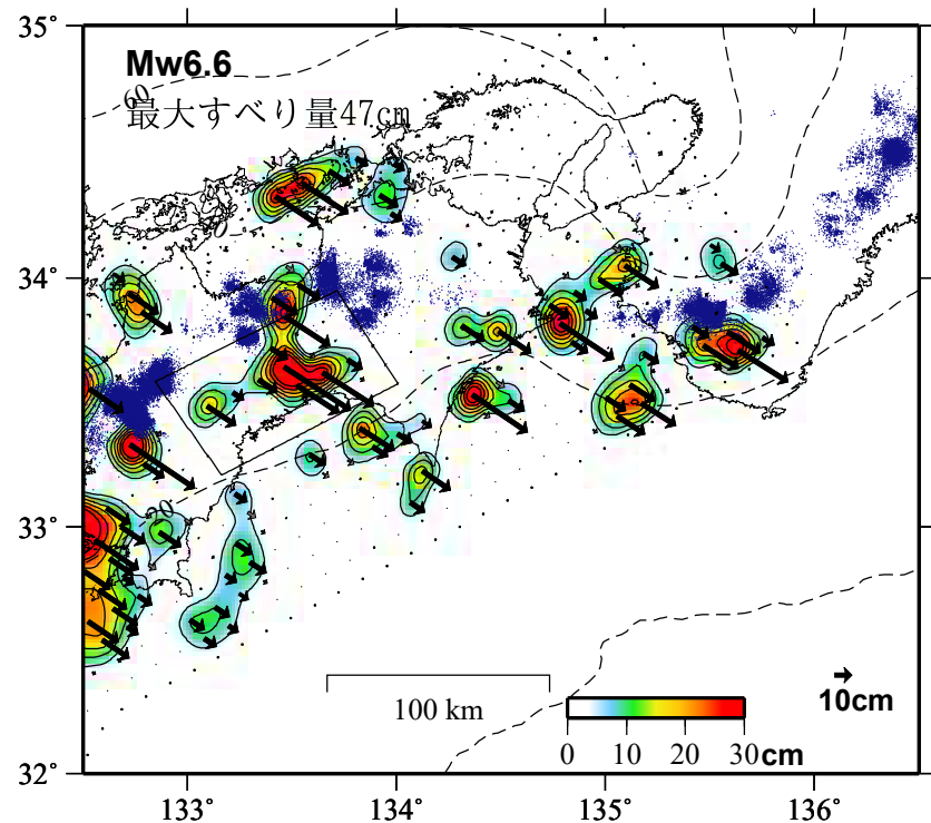
推定すべり分布 (2019-01-01/2024-02-08)
