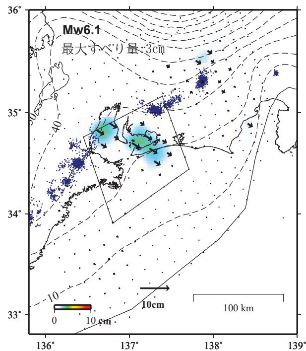
推定すべり分布 (2022-01-01/2023-12-21)
