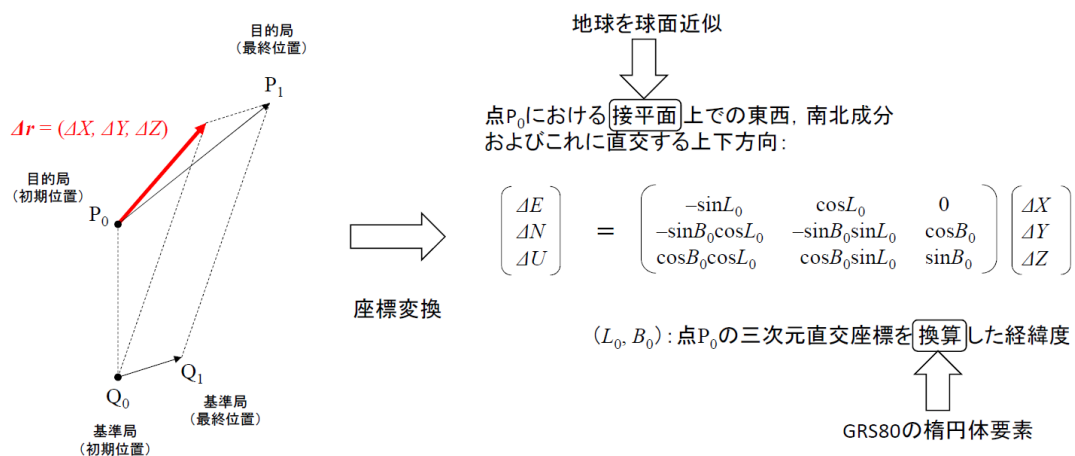
図-1 基線ベクトルの成分変化量
