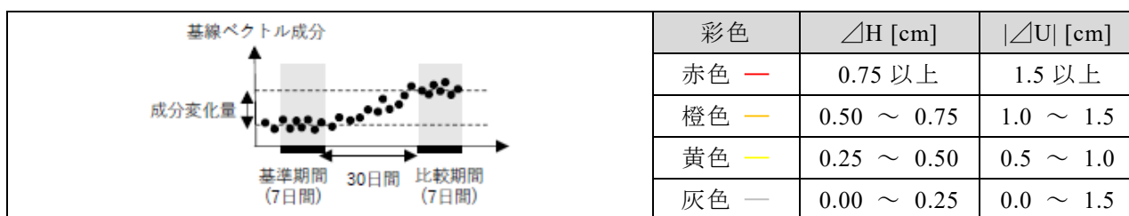
図-2 観測期間と閾値（彩色規準）
