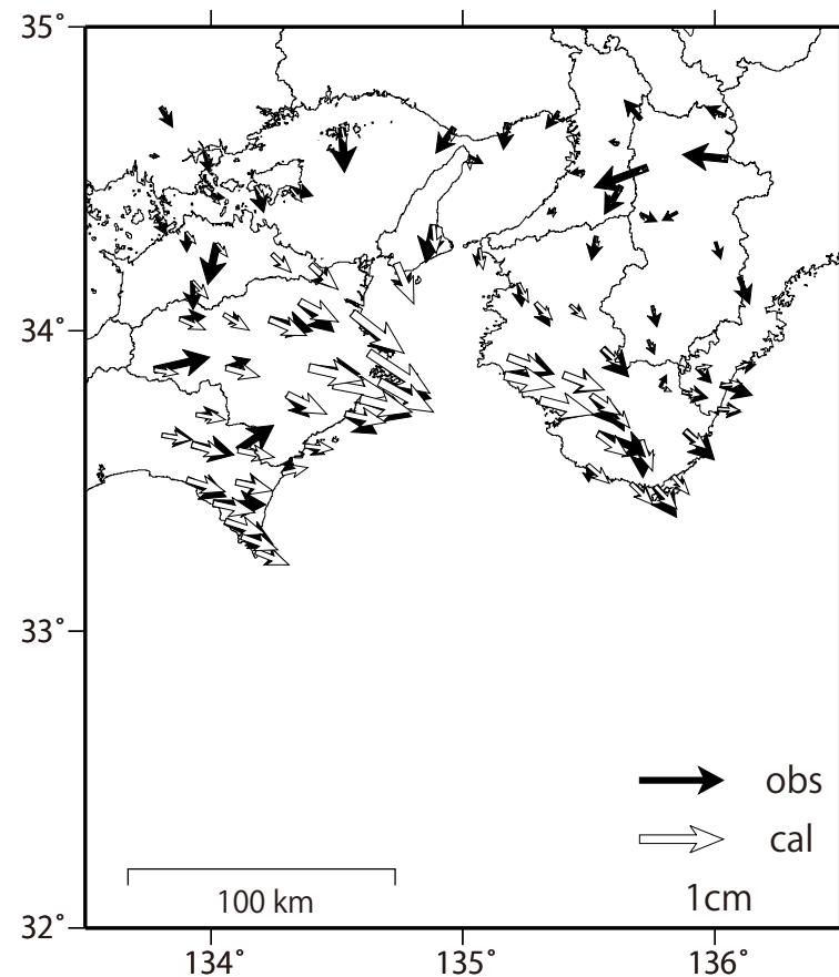
観測値(黒)と計算値(白)の比較 (2020/6/1-2022/2/10)
