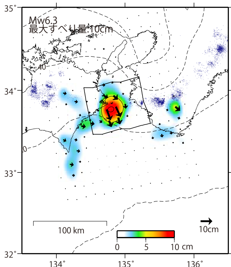
推定すべり分布 (2020/6/1-2022/2/10)
