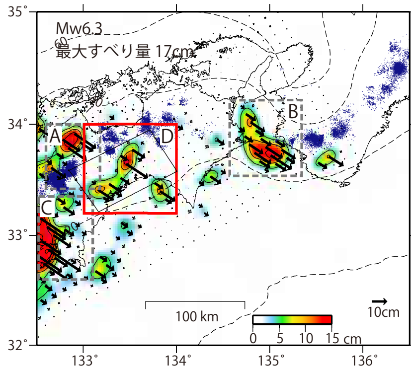
推定すべり分布 (2019/1/1-2021/12/2)
