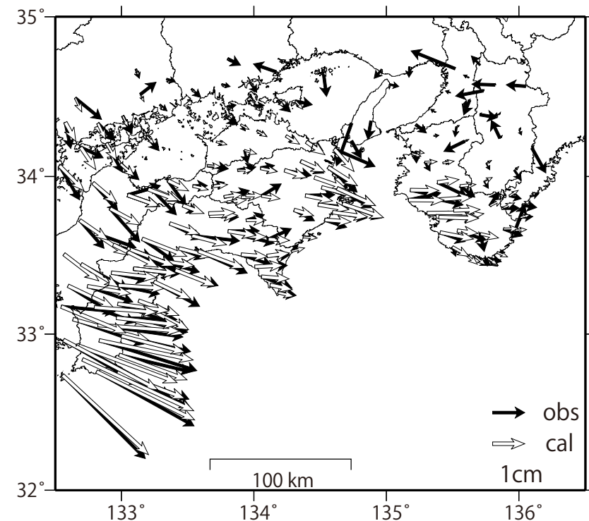
観測値(黒)と計算値(白)の比較 (2019/1/1-2021/12/2)
