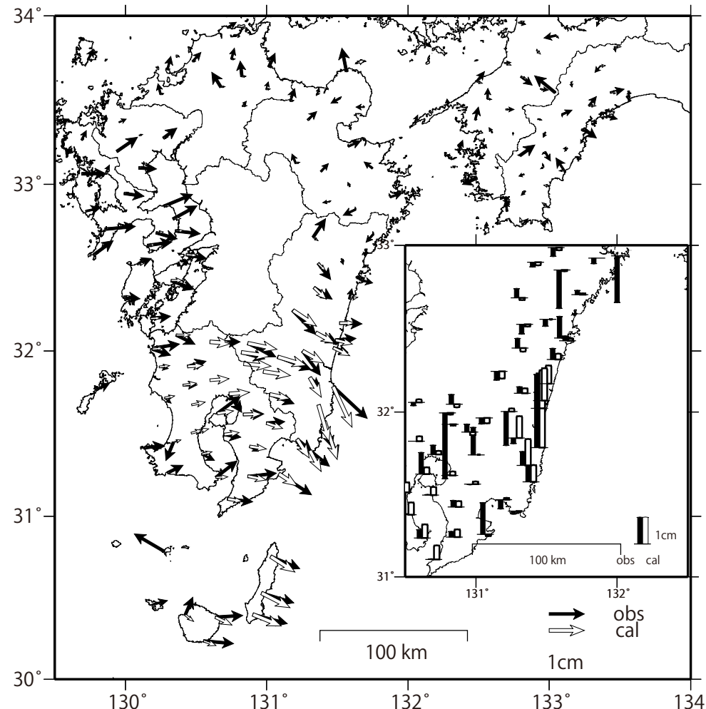
観測値（黒）と計算値（白）の比較 (2020/6/1-2021/12/3)
