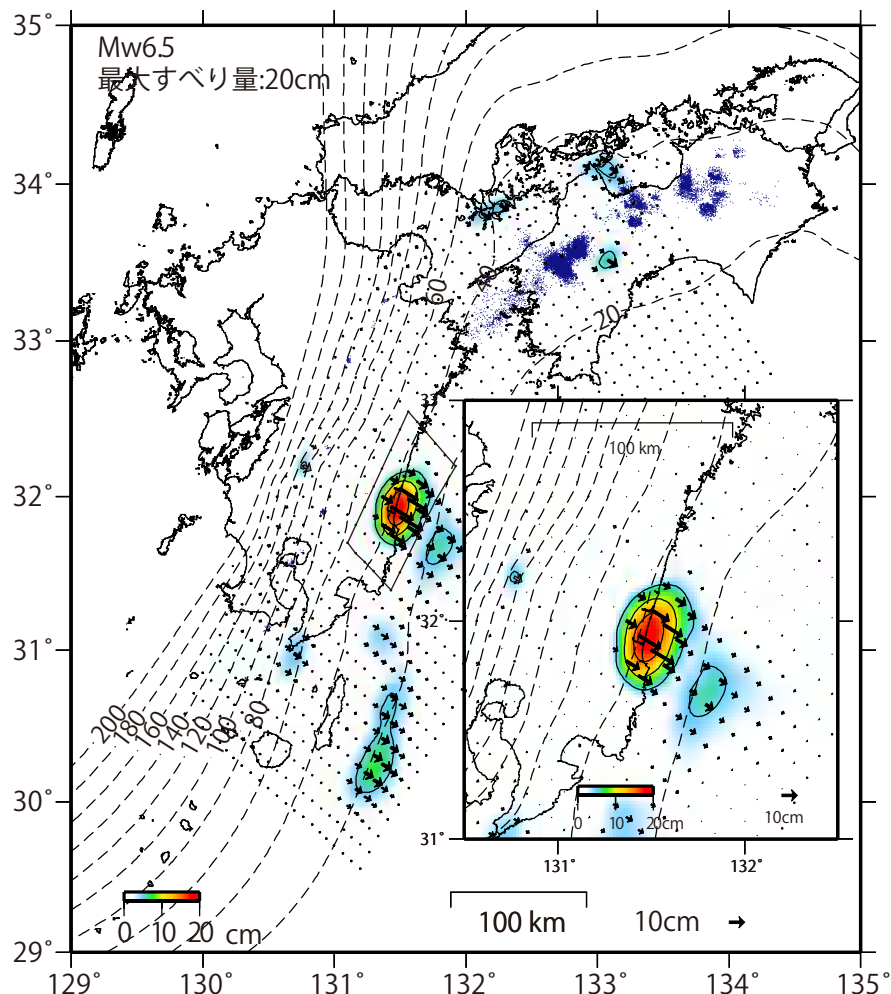
推定すべり分布 (2020/6/1-2021/12/3)
