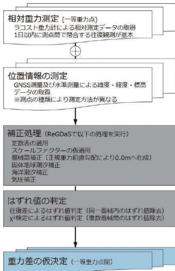
図-5 相対重力測定 of データ処理の流れ
