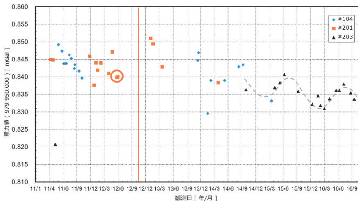
図-3 筑波 FGS の絶対重力値の時系列変化. 橙の丸印は筑波 FGS における JGSN2016 の成果値 (2012 年 6 月の値), 橙の縦線は重力鉛直勾配の測定日 (2012 年 10 月), 点線は 2014 年 9 月～2016 年 9 月の FG5 (#203) の測定に対する重力変化の近似曲線.
