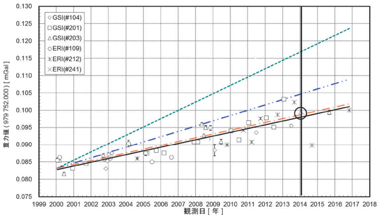
図-4 御前崎 FGS の絶対重力値の時系列変化。黒丸は御前崎 FGS での JGSN2016 の成果値（2014 年 1 月の値）、黒の縦線は重力鉛直勾配の測定日（2014 年 1 月）。黒の実線は実測値から推定した重力変化の近似直線、橙の破線は、御前崎 FGS での実測重力鉛直勾配に基づいてブーゲー勾配を仮定し、御前崎の沈降速度から重力変化を推定した近似直線、青の破線はブーゲー勾配を -1.967 \mu\text{Gal}/\text{cm} と仮定した重力変化の近似直線、緑の点線はフリーエア勾配を -3.086 \mu\text{Gal}/\text{cm} と仮定した重力変化の近似直線。
