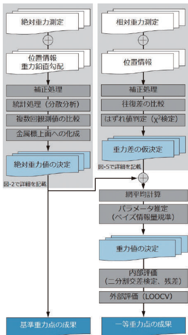
図-1 JGSN2016 構築の流れ
