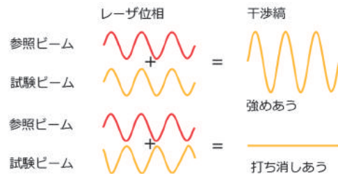
図-3 干渉縞（フリンジ）発生の様式図
