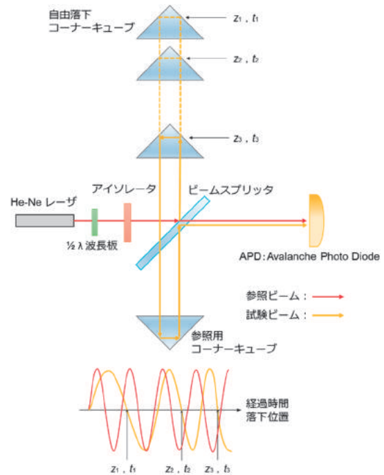
図-2 FG5 で用いるマイケルソン干渉計の概要
