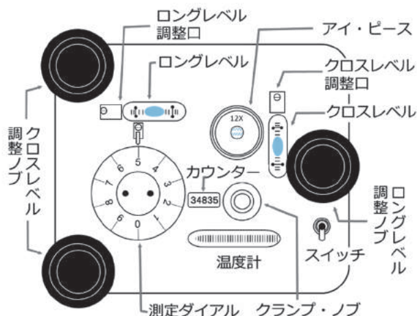
図-19 ラコスト重力計の概略図（上面から見た場合）
