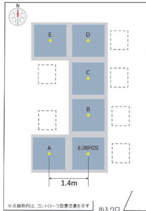
図-12 石岡測地観測局重力測定室見取り図
