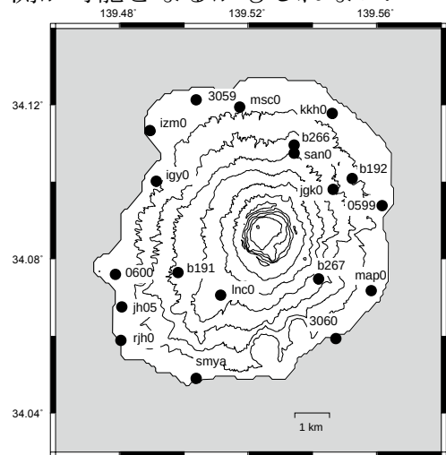
図1. シミュレーションの観測点配置
