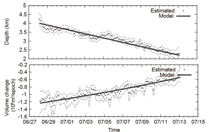
図2. シミュレーション結果. 実線がモデル値、点が推定値、点線が推定値の 95%信頼区間を表す。
