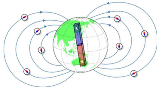
地球は大きな磁石
