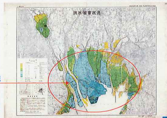
伊勢湾台風洪水被害状況図
