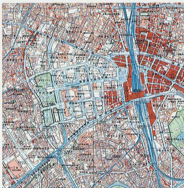
1万分1地形図「新宿(平成11年)」部分
