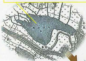
5万分1地形図 「鹿島(潮来)(明治36年)」部分
