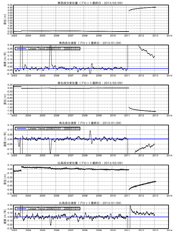
三隅 (950388) -- 矢本 (960549) 間の成分変位と速度グラフ
