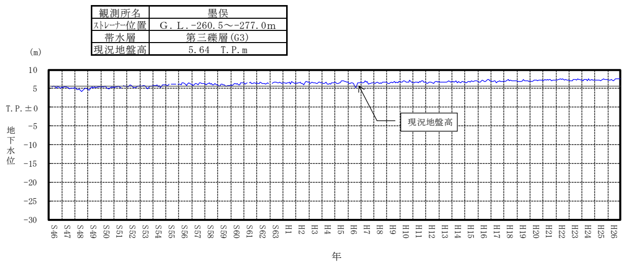
付図-2(11) 地下水位変動（墨俣）
