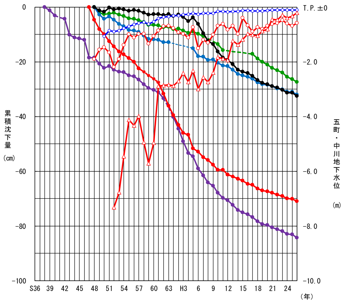
図ー 7 水準点の累積沈下量（過去5年間の累積沈下量が大きい5水準点） と地下水位観測所の年平均地下水位
