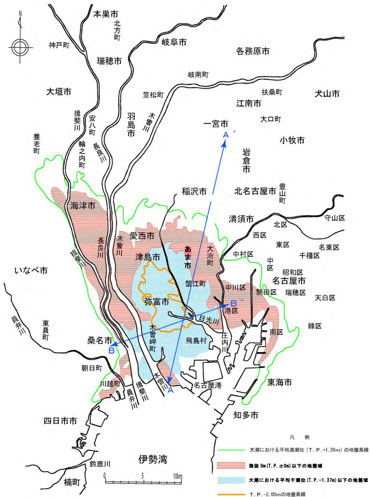
図-9 海拔ゼロメートル地帯
