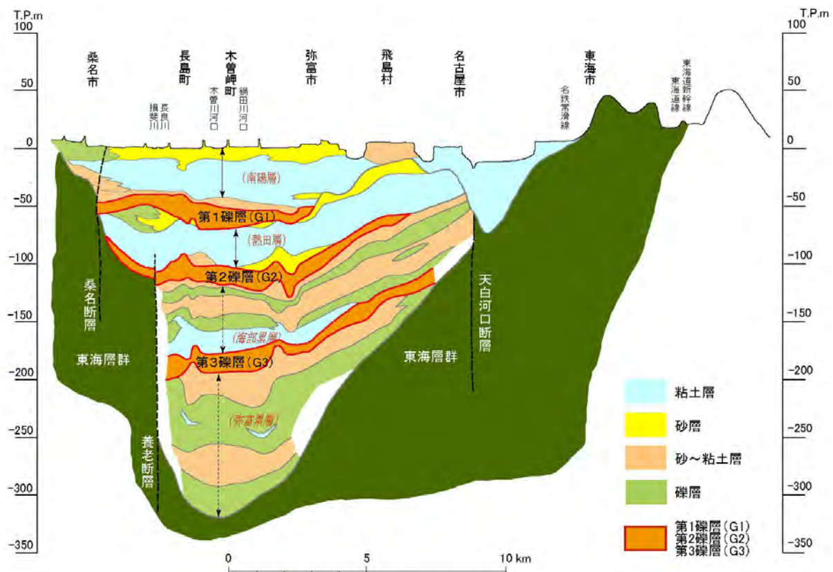
図－4(2) 濃尾平野の地層断面(A-A' 測線：桑原(1985)を一部改変) (図中の白抜き部分は、資料が少なく、累層判定が困難な部分)
