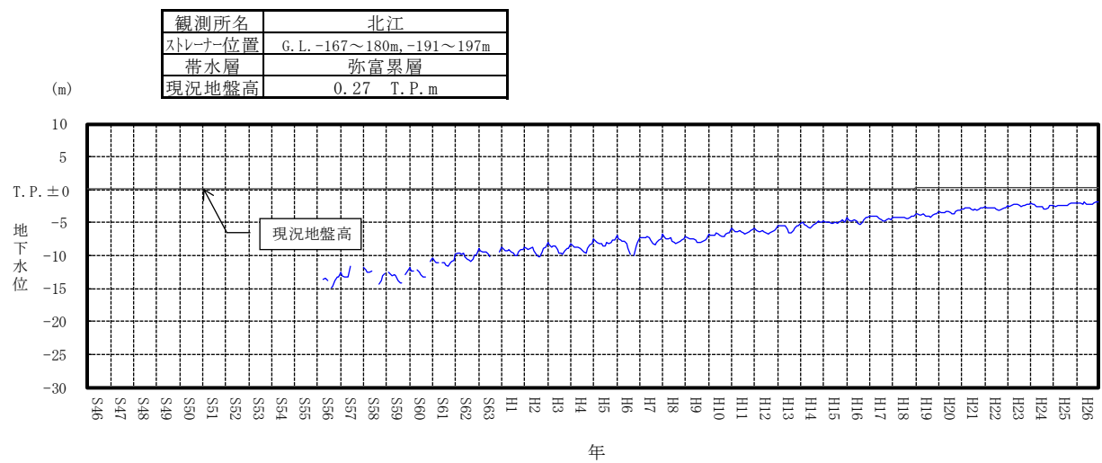
付図-2(15) 地下水位変動（北江）
