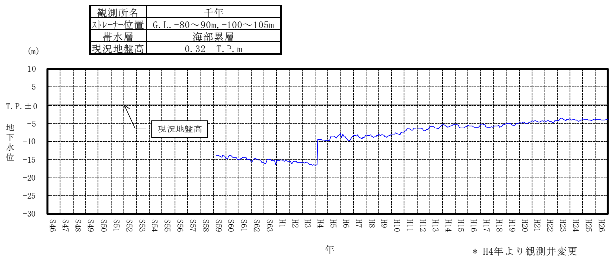
付図-2(14) 地下水位変動（千年）
