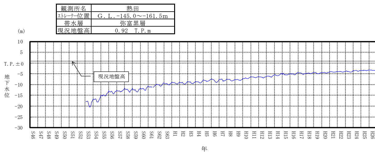
付図-2(17) 地下水位変動（熱田）
