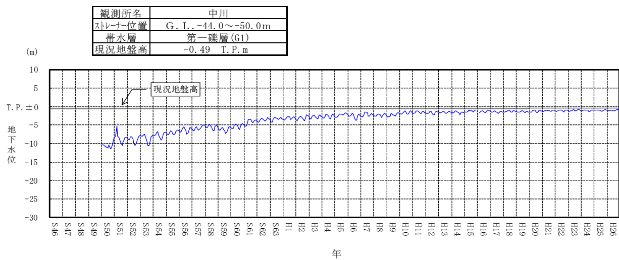
付図-2(18) 地下水位変動（中川）
