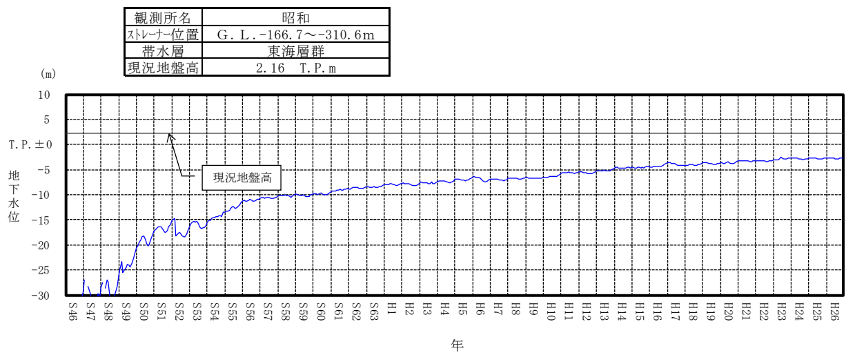
付図-2(16) 地下水位変動（昭和）
