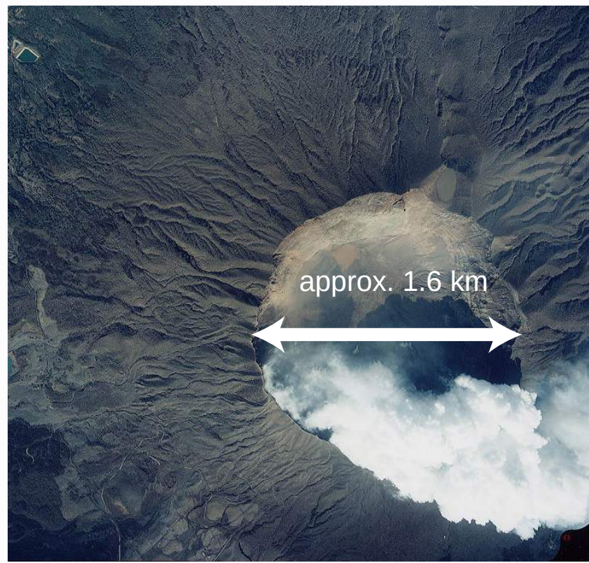
Fig. 2 Summit caldera
