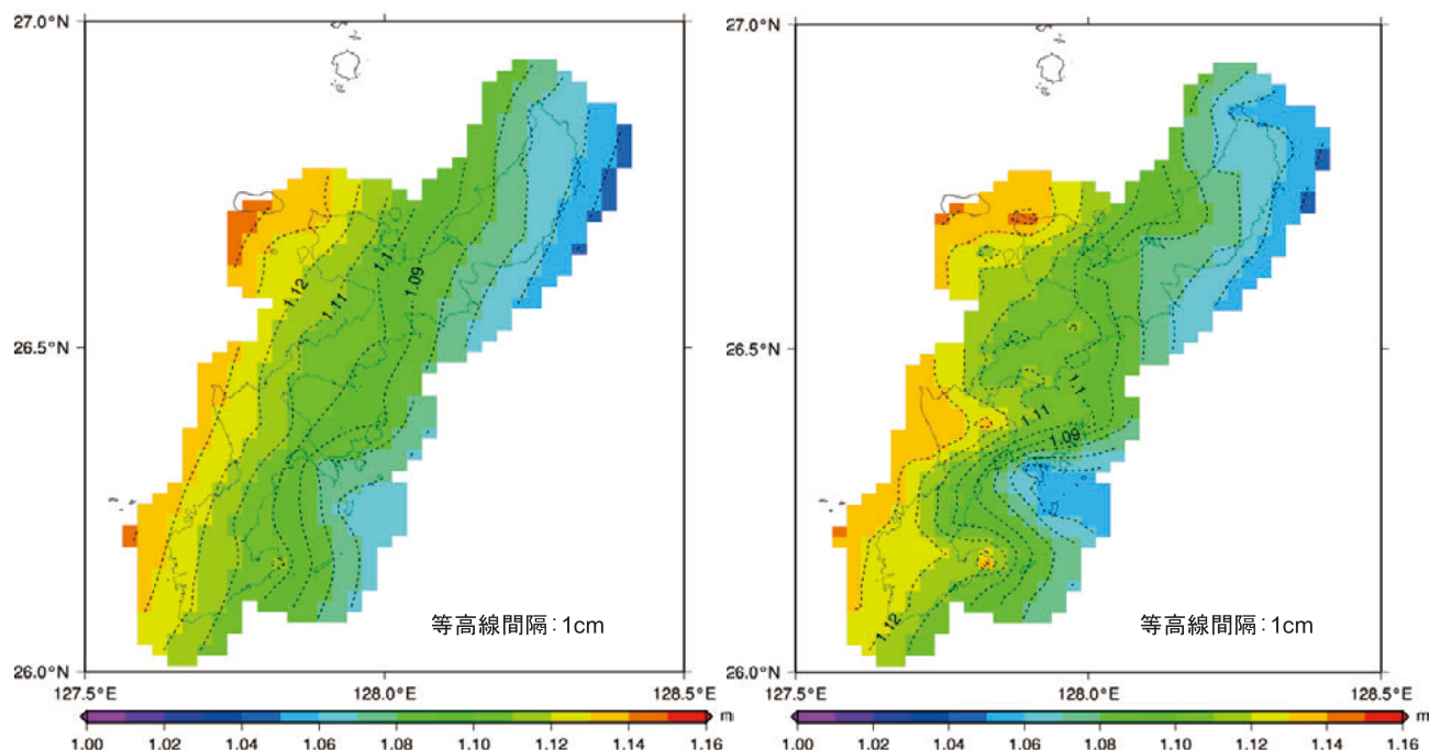
図-18 ジオイド補正モデル（左：greenspline プログラムにより作成，右：surface プログラムにより作成）
