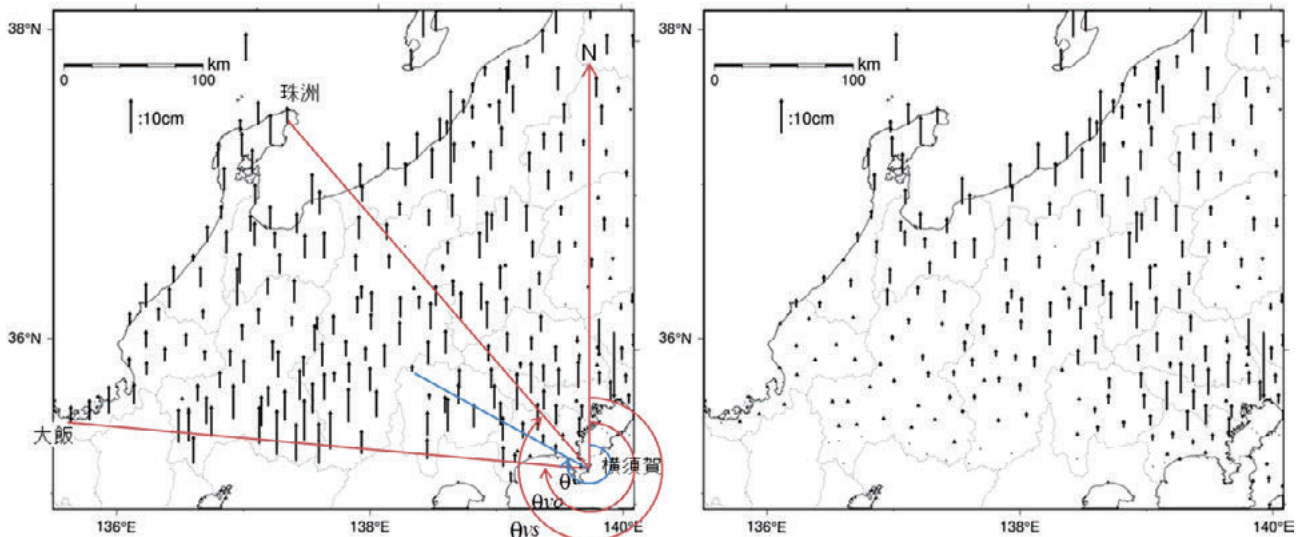
図-2 電子基準点の楕円体高の改定量分布（左：調整前の成果改定量；電子基準点「横須賀」を基点とする各点の方位角が \theta ，右：調整後の成果改定量；調整地域では北東端から南西端に向かって次第に更新量が小さくなる）
