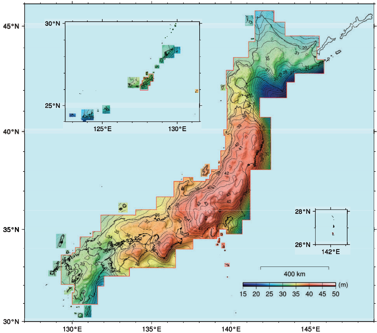
図-11 「日本のジオイド 2011」(Ver. 1) の陰影段彩表現 (等高線の間隔は 0.2m, 適用: 赤枠内「日本のジオイド 2011」, その他の地域「日本のジオイド 2000」Ver.5)
