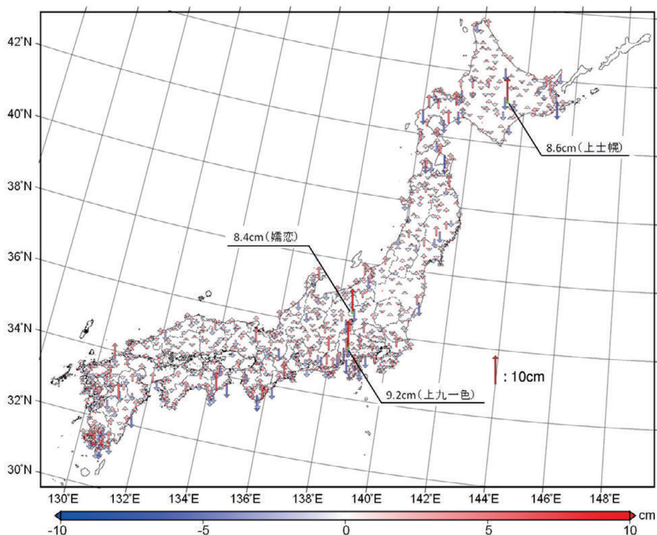
図-5 ジオイド高データとジオイド・モデルとのジオイド高の差
