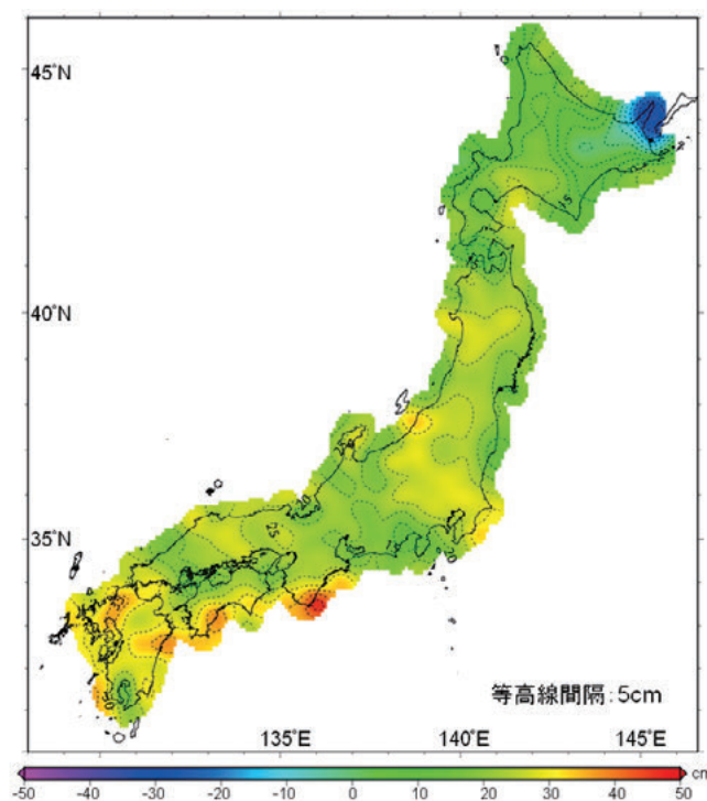
図-10 全国のジオイド較差モデル
