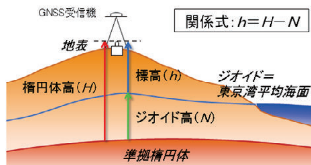
図-1 楕円体高、標高及びジオイド高の関係
