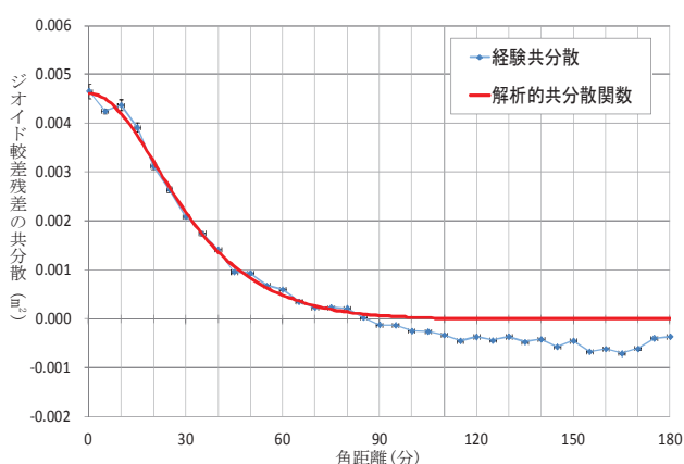
図-8 「日本のジオイド 2011」の構築に用いられるジオイド較差残差の経験共分散と解析的共分散関数
