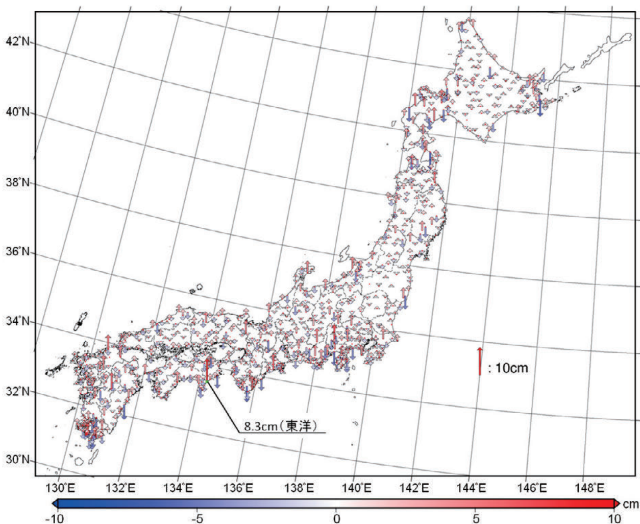
図-14 「日本のジオイド 2011」構築に使用したジオイド高データと「日本のジオイド 2011」のジオイド高の差
