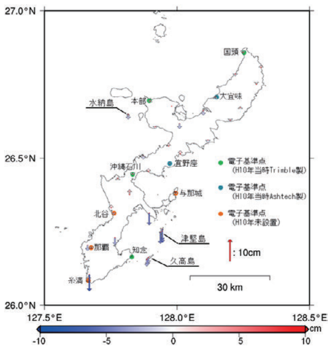
図-17 ジオイド高データと電子基準点のみで構築したジオイド・モデルによるジオイド高との差
