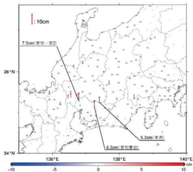
図-3 楕円体高の調整前と調整後のジオイド高データと ジオイド・モデルの較差（絶対値）の差
