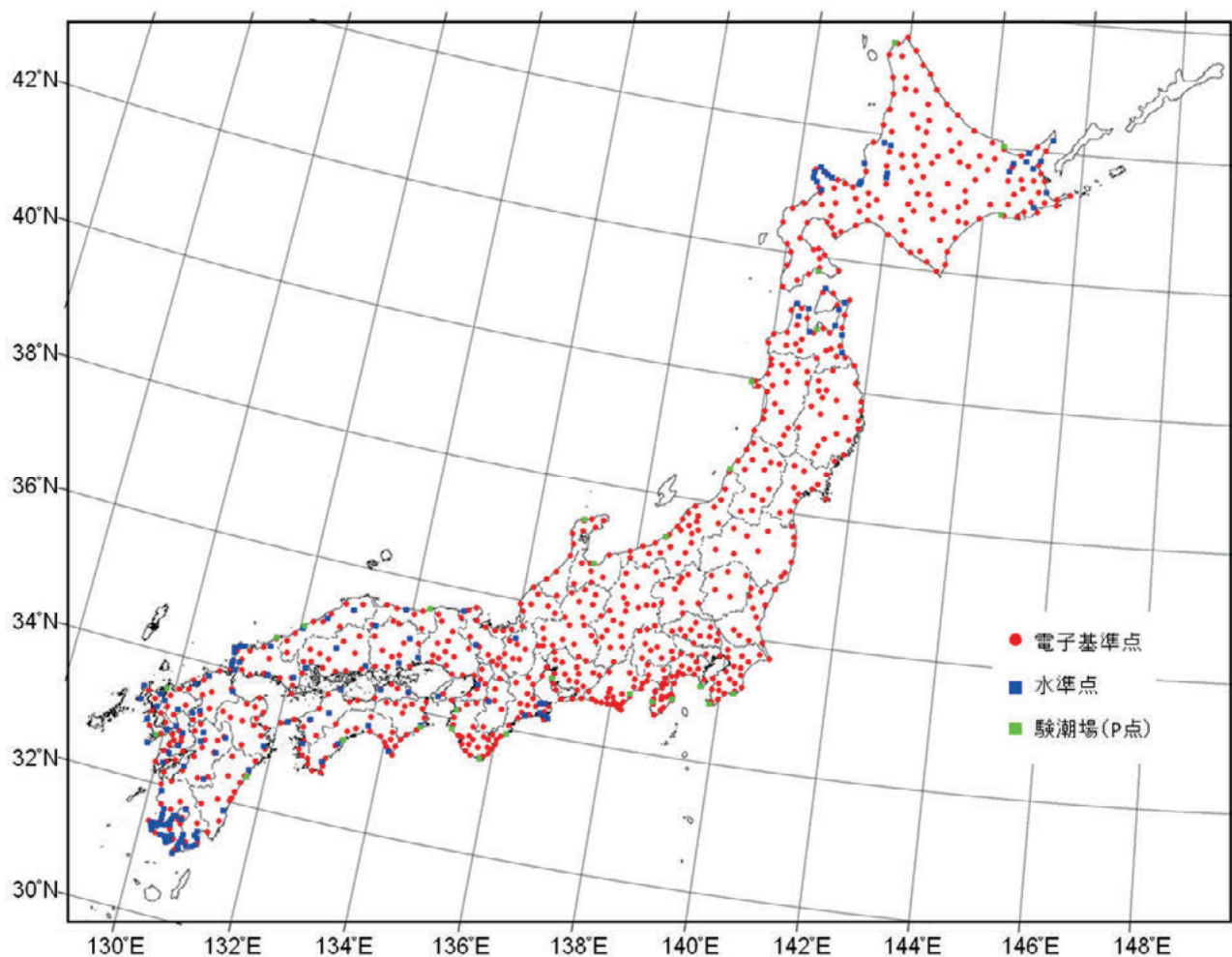
図-4 「日本のジオイド 2011」の構築に使用するジオイド高データの分布
