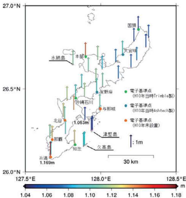
図-16 ジオイド高データと JGEOID2008 の差
