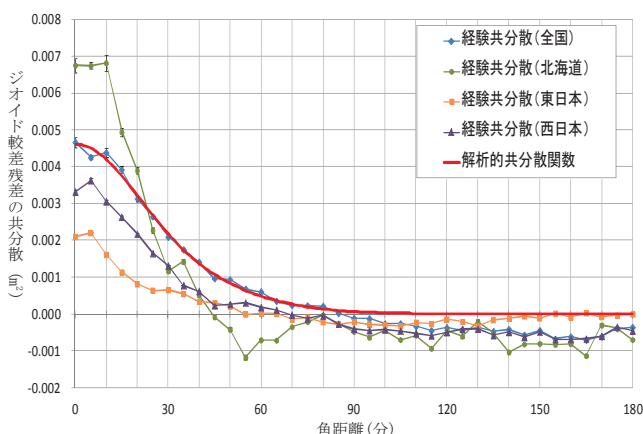
図-9 地域別の経験共分散と決定した解析的共分散関数
