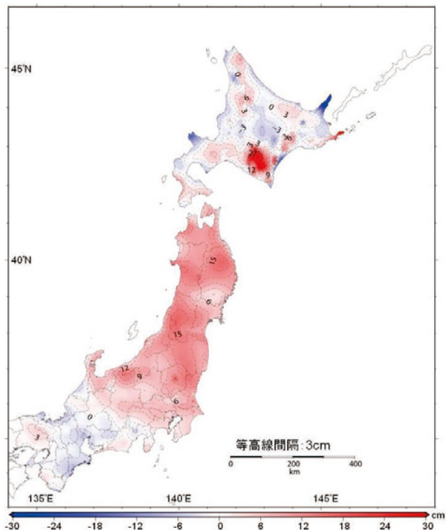
図-13 「日本のジオイド 2011」と「日本のジオイド 2000」 のジオイド高の差
