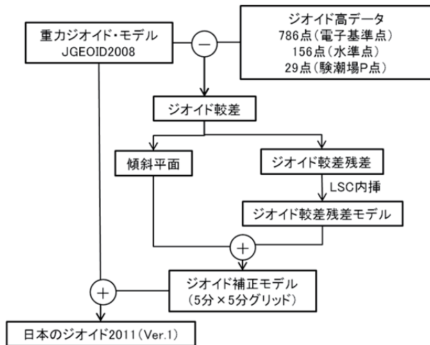
図-6 「日本のジオイド 2011」(Ver.1) (沖縄島を除く) を構築する処理の概念図
