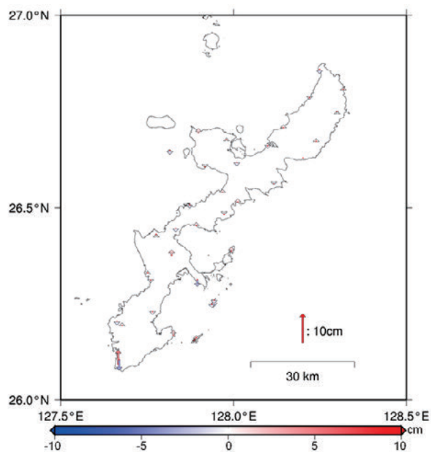
図-19 構築に使用したジオイド高データとジオイド・モデルによるジオイド高の差
