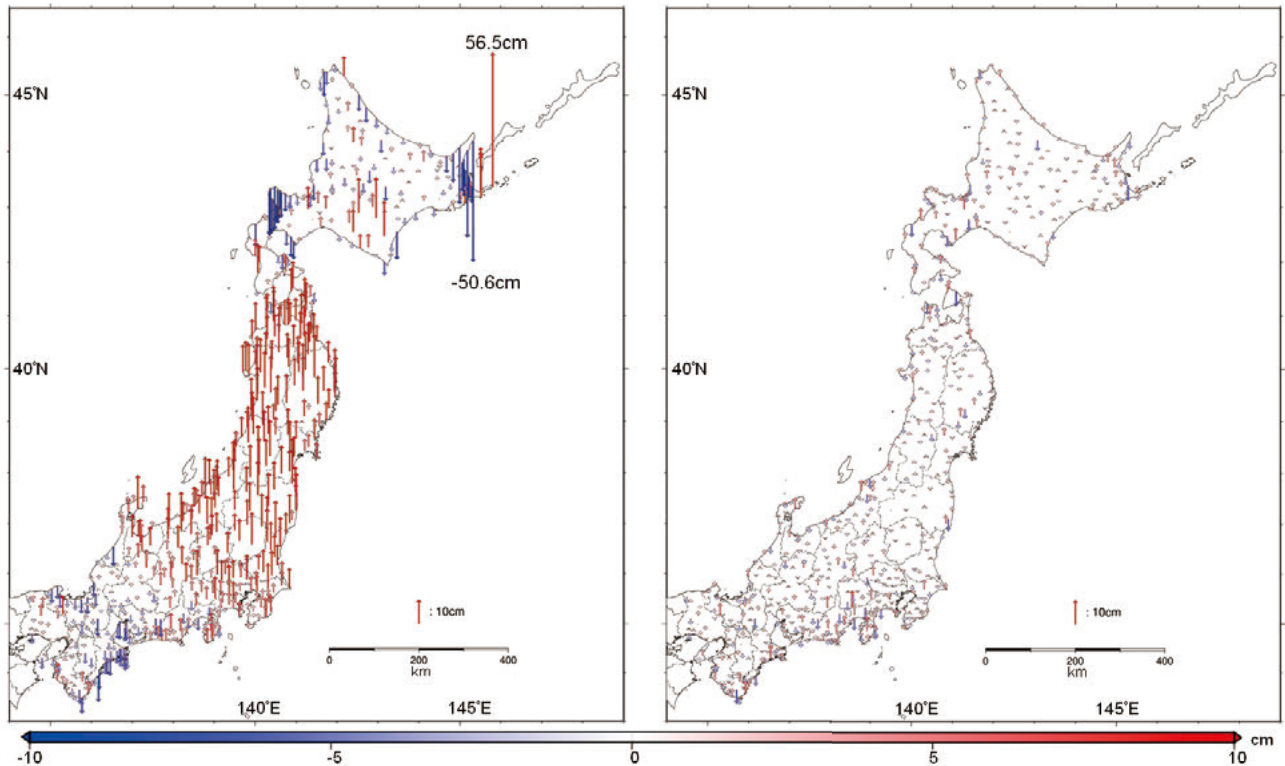
図-12 「日本のジオイド 2011」構築に使用したジオイド高データと新・旧のジオイド・モデルのジオイド高の差 (左：日本のジオイド 2000, 右：日本のジオイド 2011)
