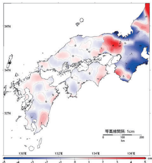
図-15 全国モデルと「日本のジオイド 2011+2000」の差
