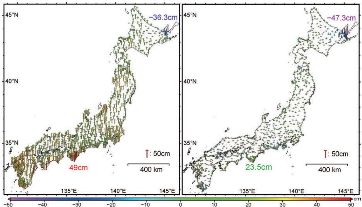
図-7 (左) JGEOID2008 とジオイド高データのジオイド較差, (右) JGEOID2008 とジオイド高データのジオイド較差の残差
