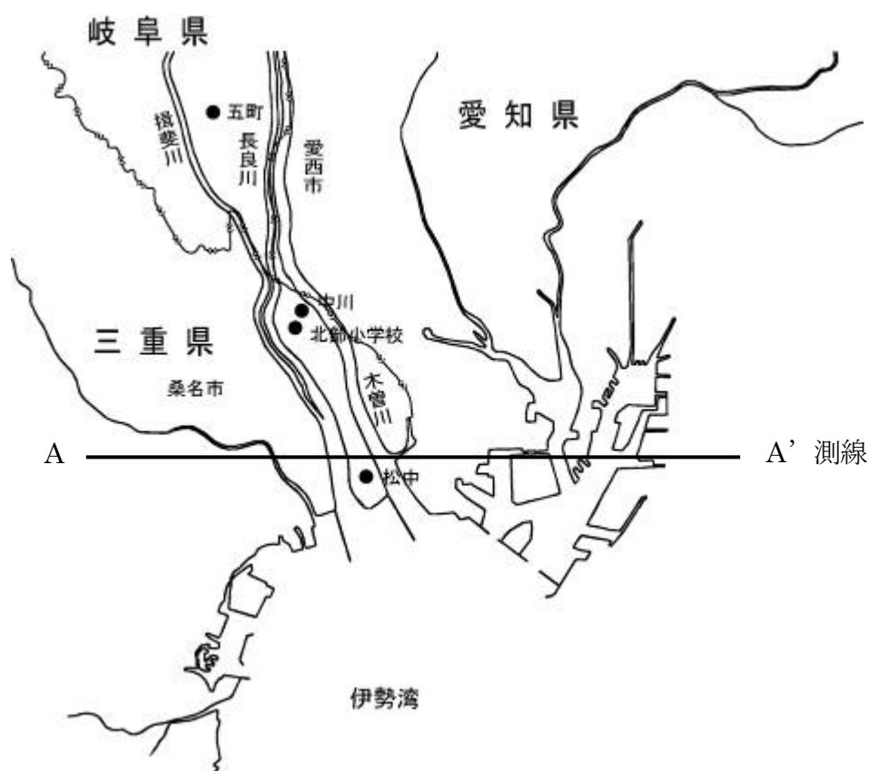
図－4(1) 地盤沈下観測所および地層断面測線の位置
