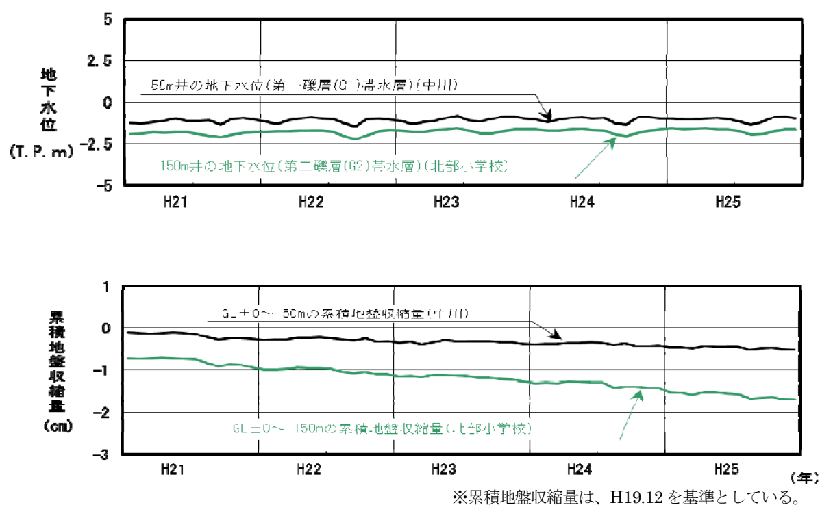
図-4(4) 中川・北部小学校観測所
