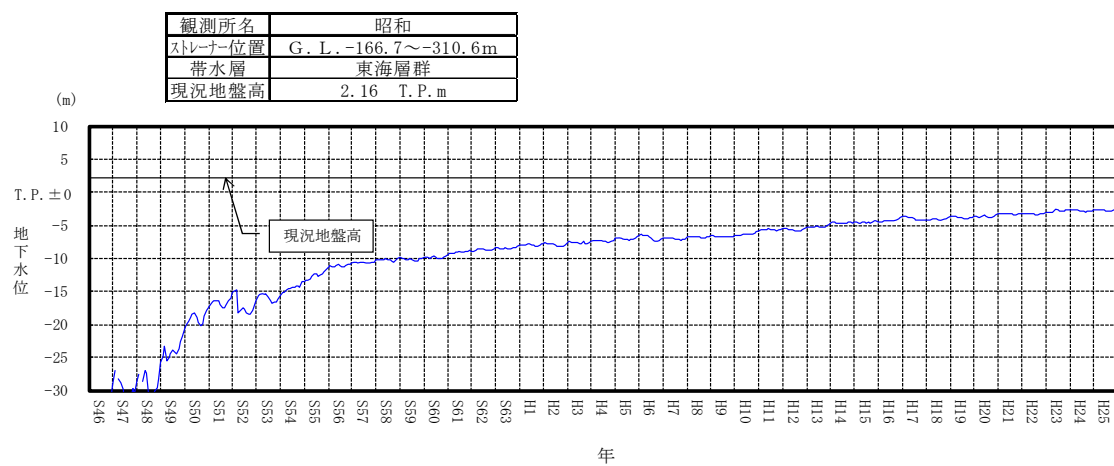
付図－2(16) 地下水位変動（昭和）
