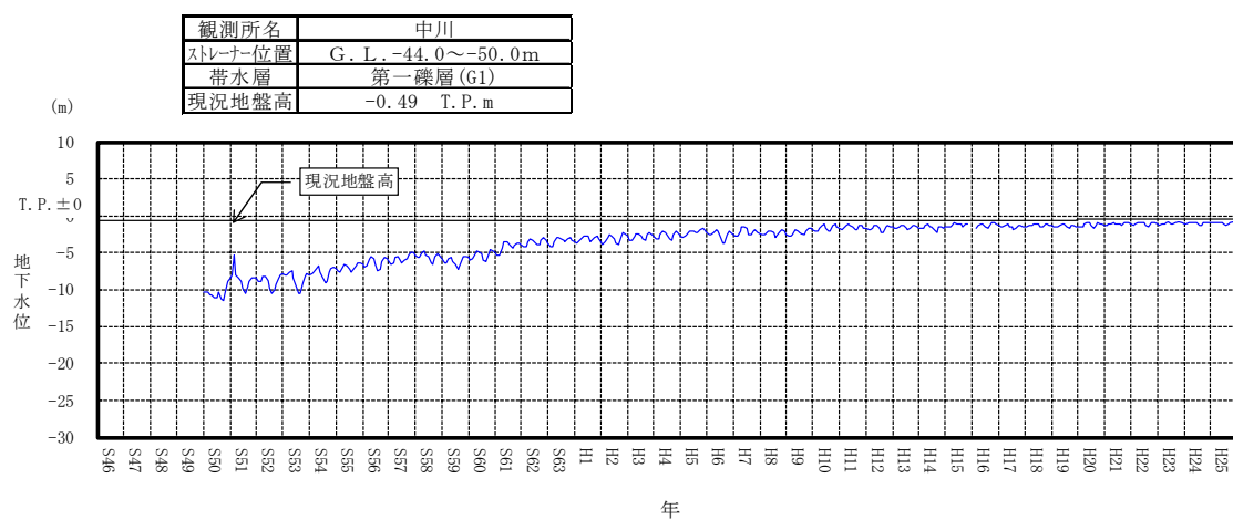
付図-2(18) 地下水位変動（中川）
