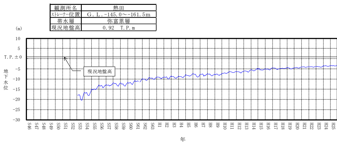
付図-2(17) 地下水位変動（熱田）
