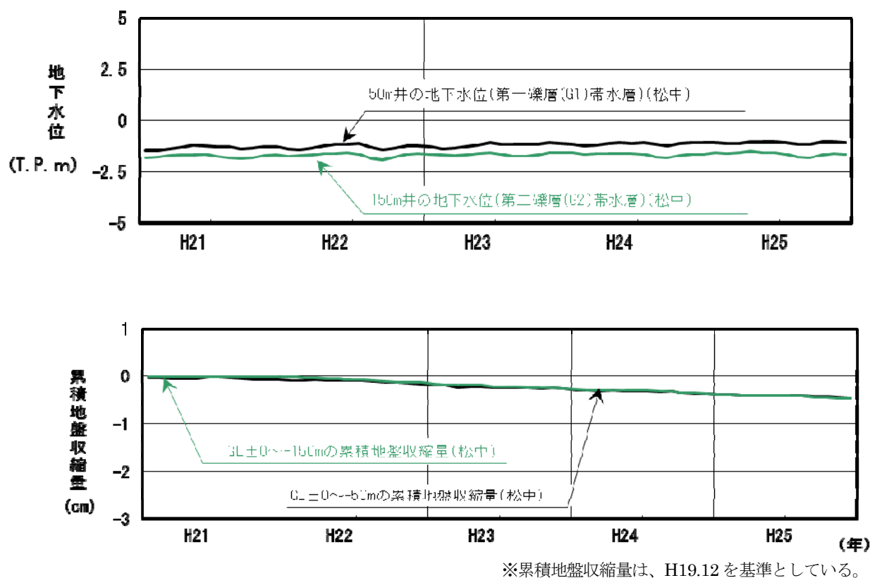
図-4(5) 松中観測所
