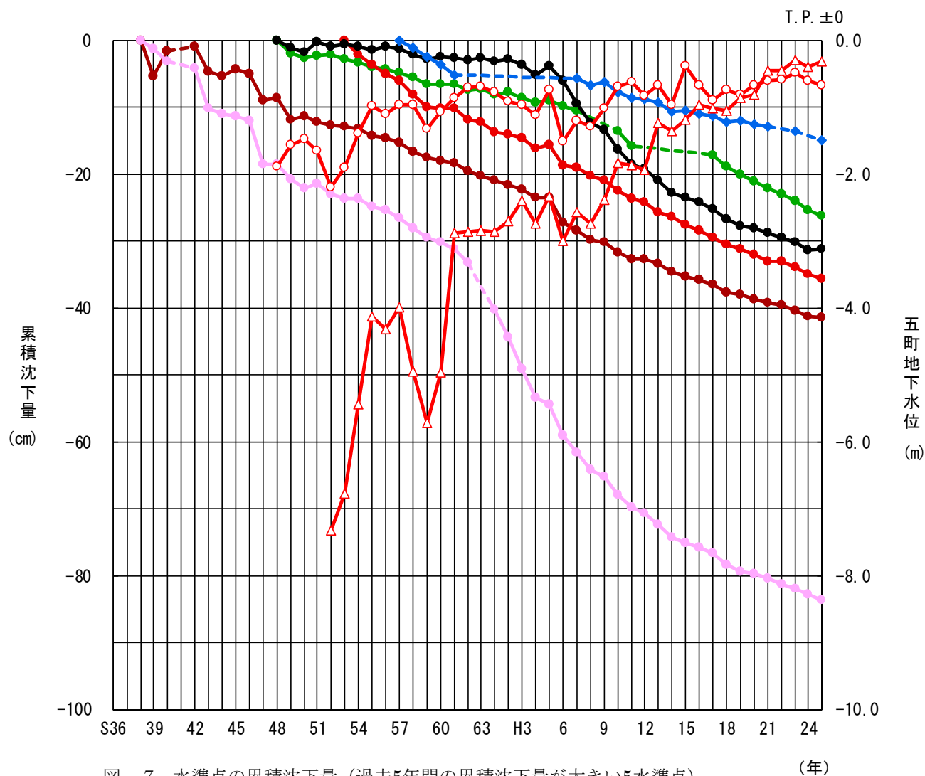
図－7 水準点の累積沈下量（過去5年間の累積沈下量が大きい5水準点） と地下水位観測所の年平均地下水位
