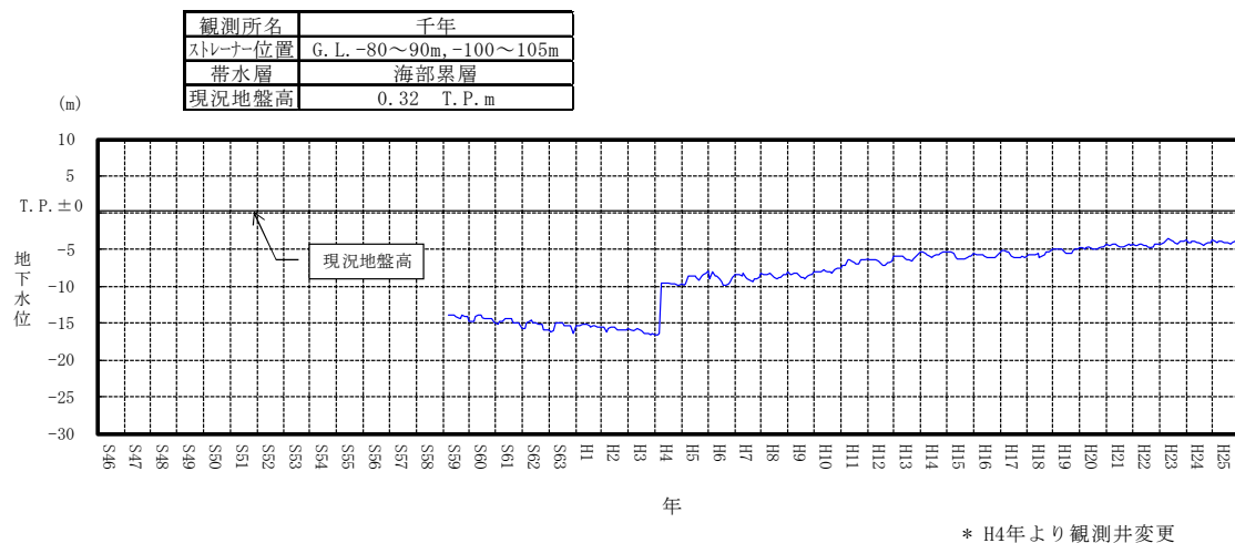
付図－2(14) 地下水位変動（千年）
