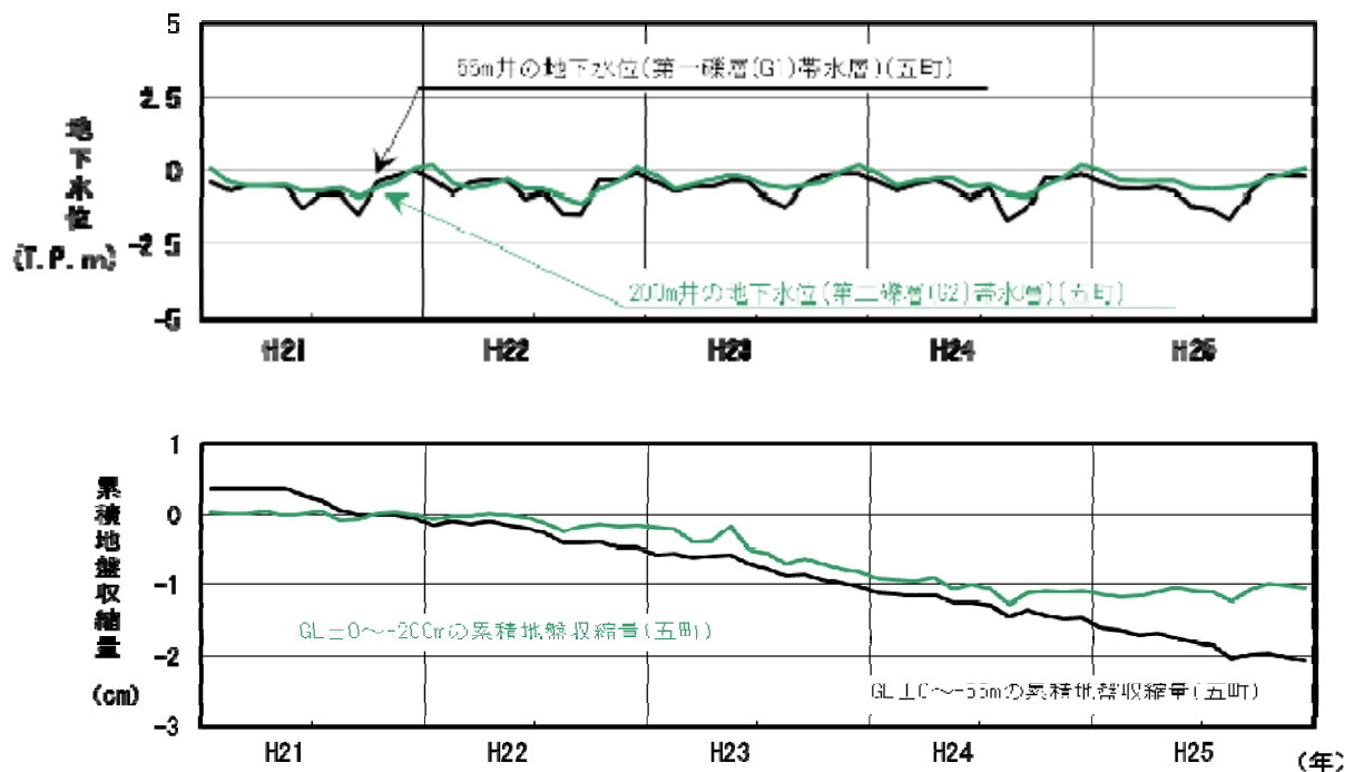
図-4(3) 五町観測所
