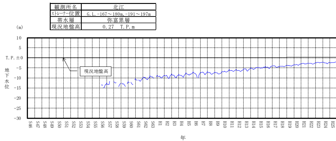
付図－2(15) 地下水位変動（北江）
