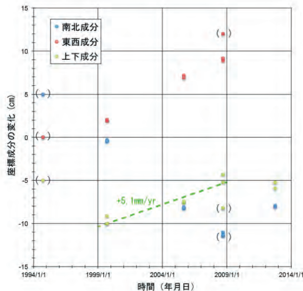
図-2 一等三角点「穂高岳」の座標変化。2012 年の東西成分は東北地方太平洋沖地震による地殻変動のためグラフの範囲外となっている。緑の点線は 1999, 2005, 2008 年の橢円体高に対する近似直線。括弧のシンボルは高度基準点測量及び高度地域基準点測量による。
