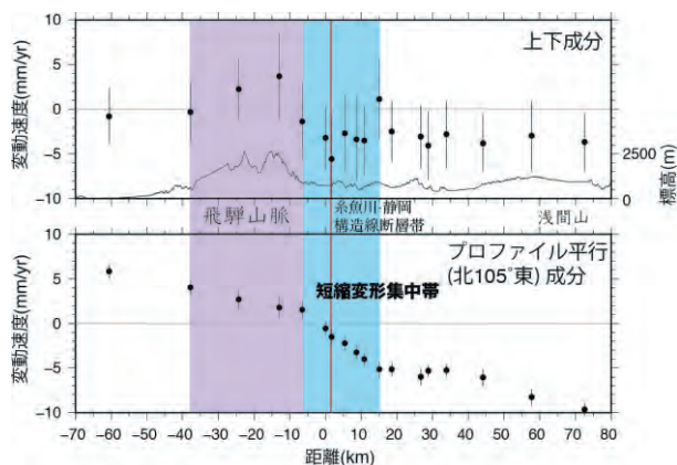
図-7 飛騨山脈立山付近を横断する測線上における変動速度プロファイル。縦棒付きの丸が変動速度、縦棒の長さが誤差 ( 3\sigma ) を表す。上下成分の実線は測線上の標高を表す。赤線は糸魚川-静岡構造線断層帯の位置。
