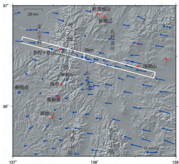
図-6 2005-2010 年の飛騨山脈及びその周辺の水平変動速度ベクトル図。穂高岳の水平変動は、1999, 2005, 2008 年の 3 回の繰り返し観測結果を示す。矩形領域は図-7 の変動プロファイルの位置を表す。
