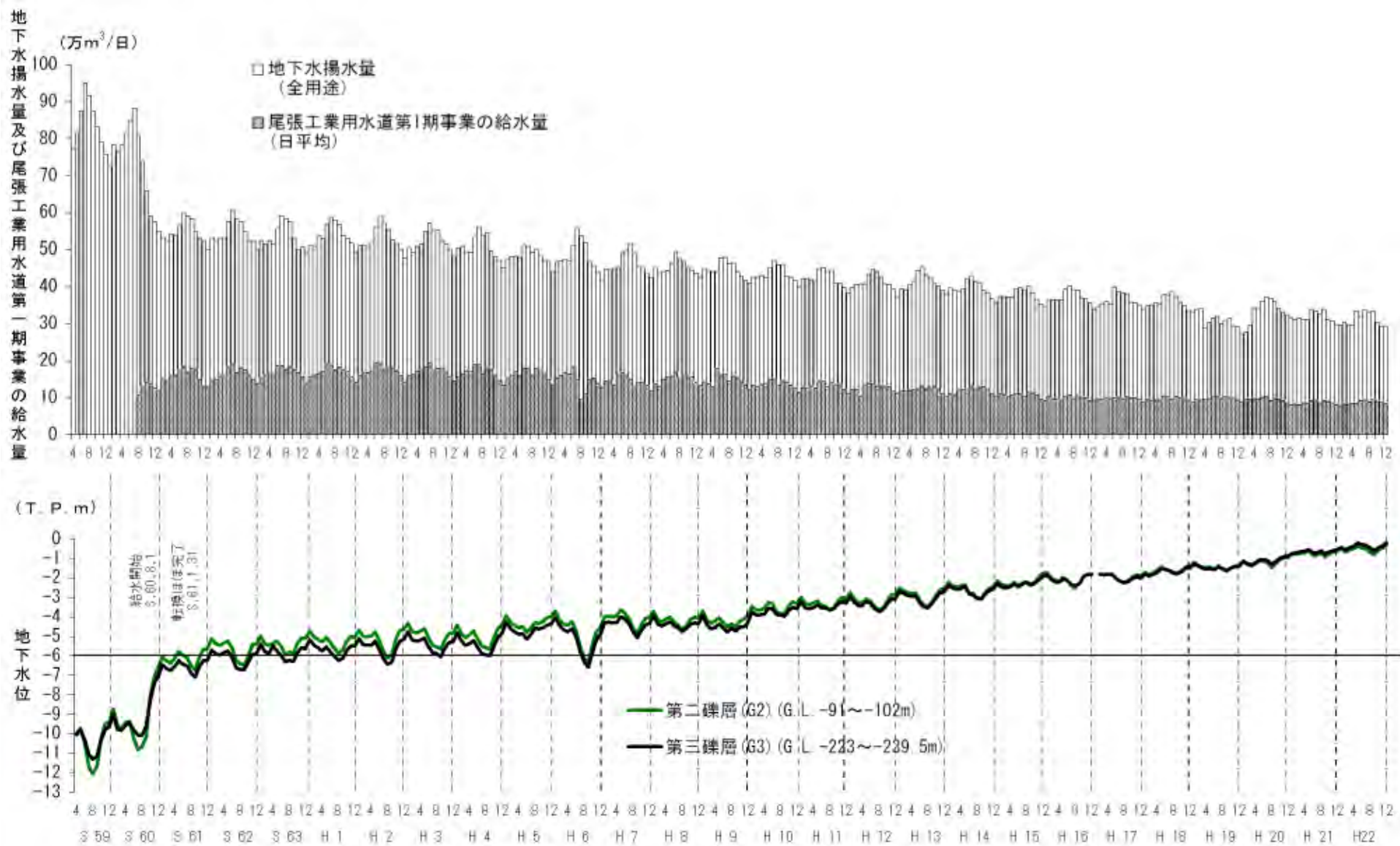
図-14 尾張工業用水道第1期事業の給水区域における給水量、地下水揚水量(全用途)、稲沢観測所の地下水位の関係
