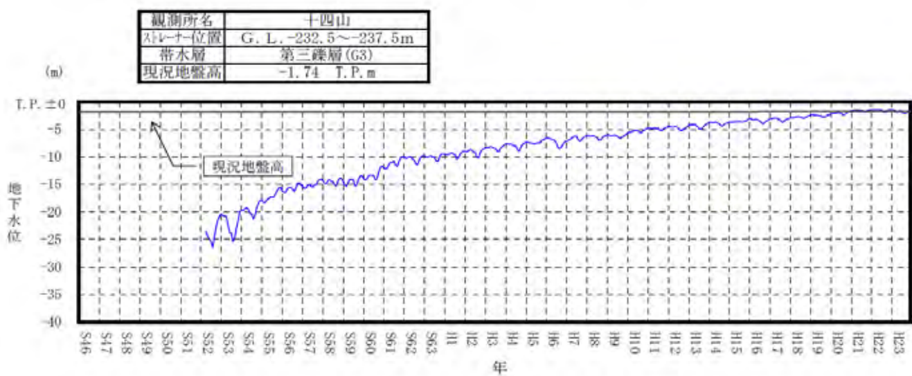
付図-2(3) 地下水位変動図 (十四山)
