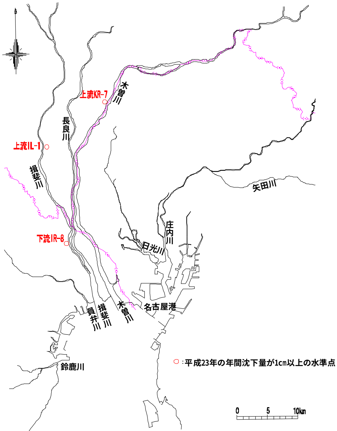
図ー1 平成 23 年における年間沈下量 1cm 以上の水準点位置
