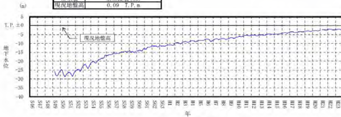
付図-2(2) 地下水水位変動図(飛島)
