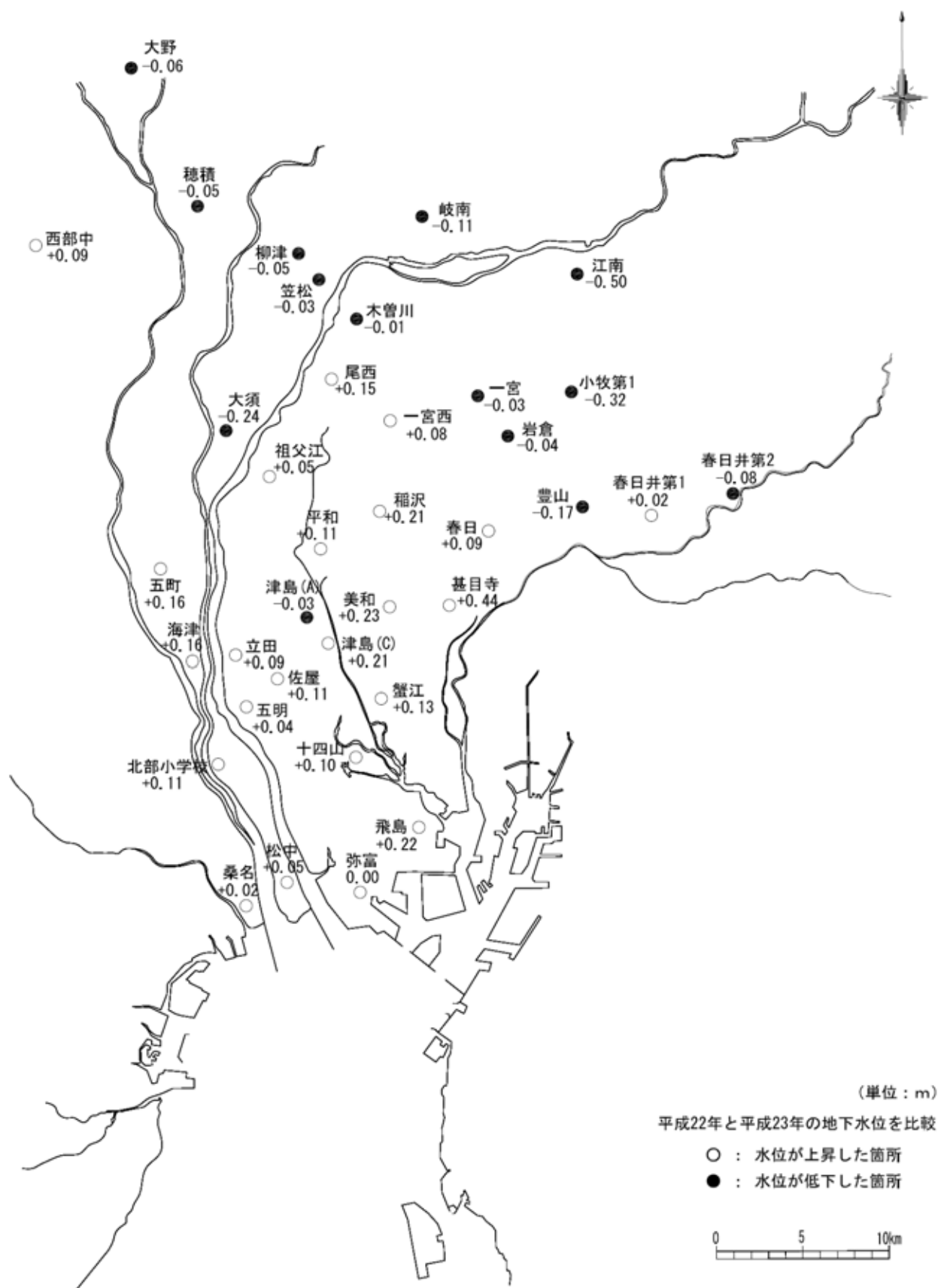
図-11(2) 年平均地下水位の変動量図 [第二礫層(G2)]
