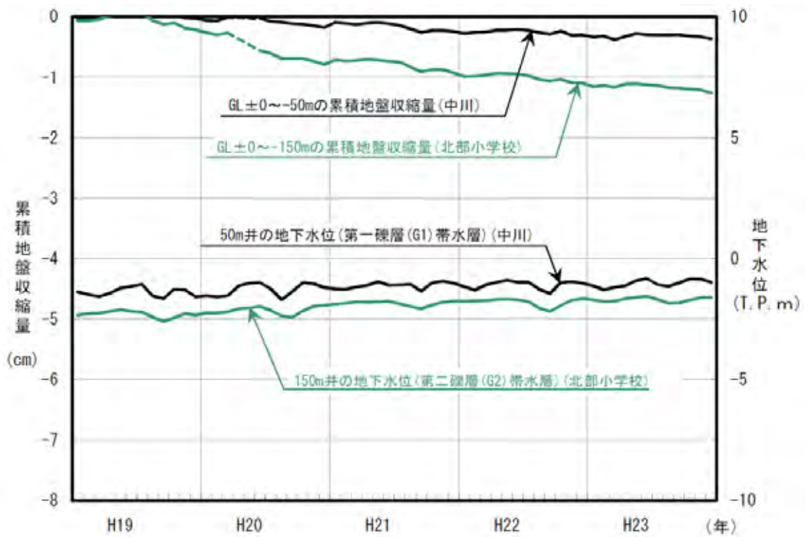
図-4(4) 中川・北部小学校観測所
