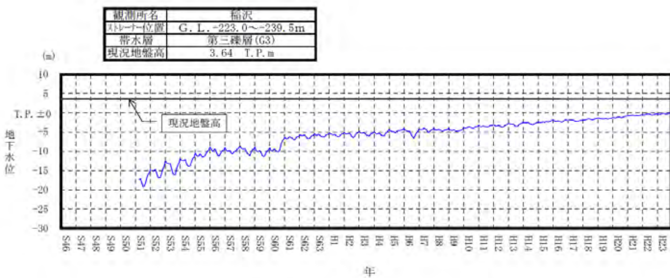
付図-2(9) 地下水位変動図(稲沢)
