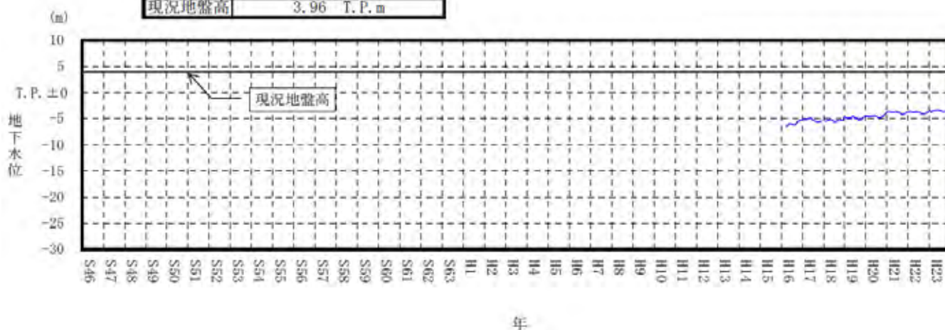
付図-2(18) 地下水位変動図（空見）
