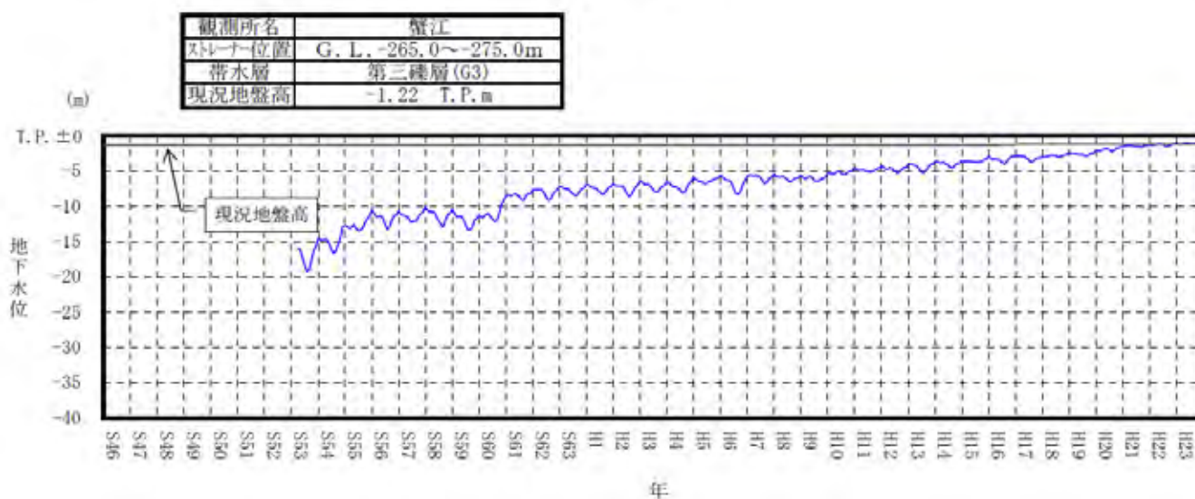
付図-2(4) 地下水位変動図(蟹江)
