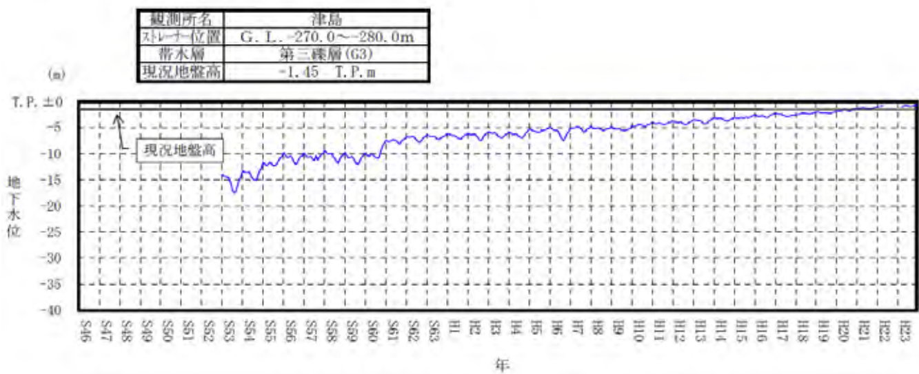
付図-2(5) 地下水位変動図(津島)
