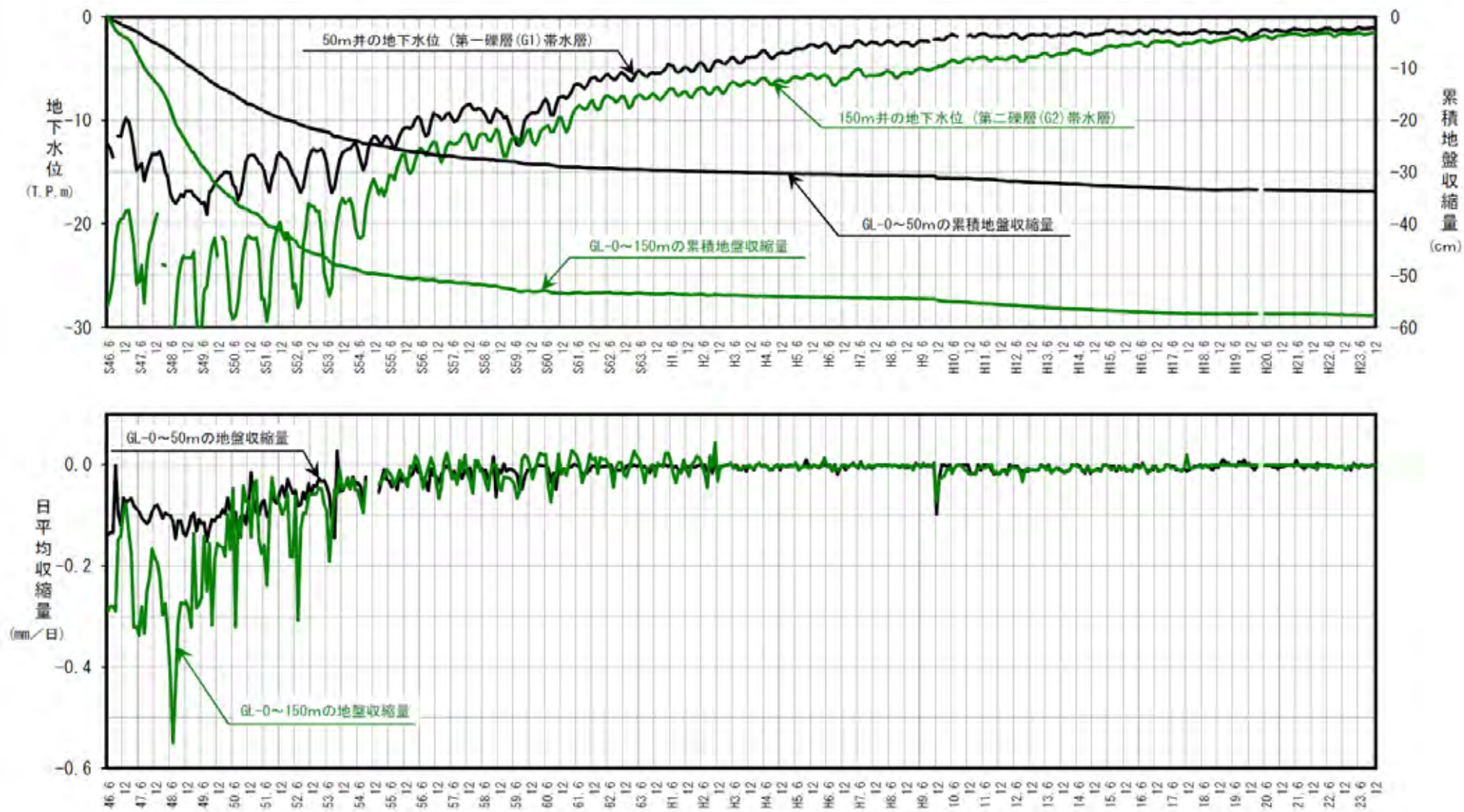
図-12 松中観測所の地下水位・地盤収縮量の変動
