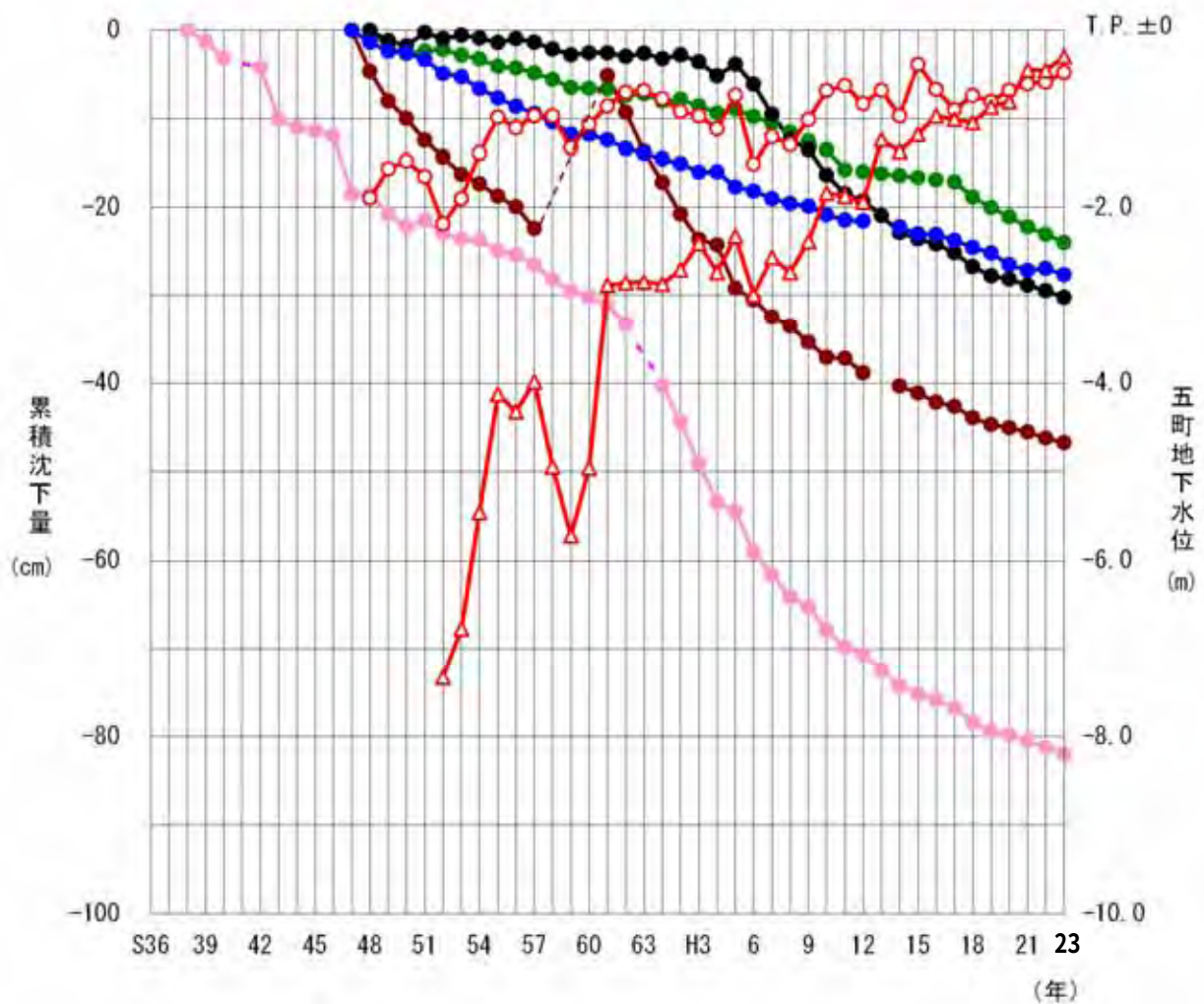
図ー7 水準点の累積沈下量（過去5年間の累積沈下量が大きい5水準点） と地下水位観測所の年平均地下水位
