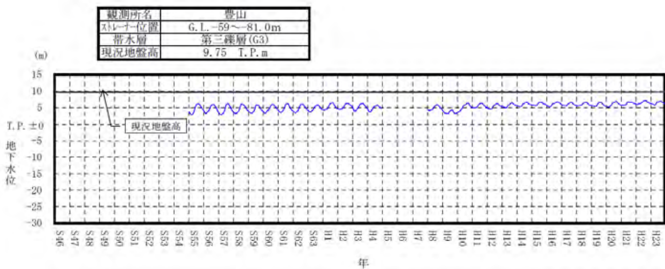
付図-2(20) 地下水位変動図 (豊山)
