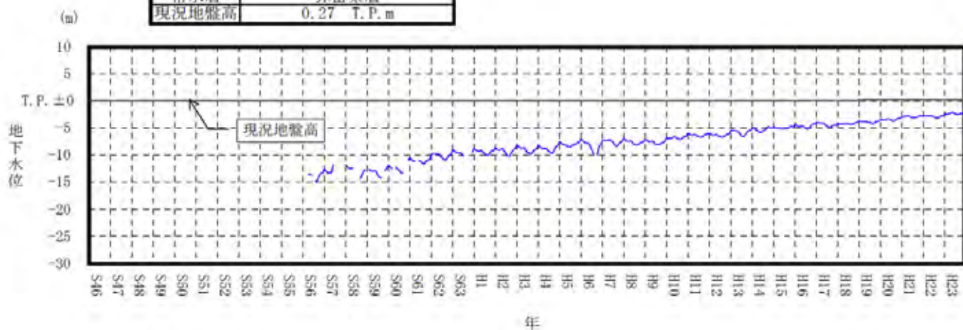
付図-2(15) 地下水位変動図 (北江)
