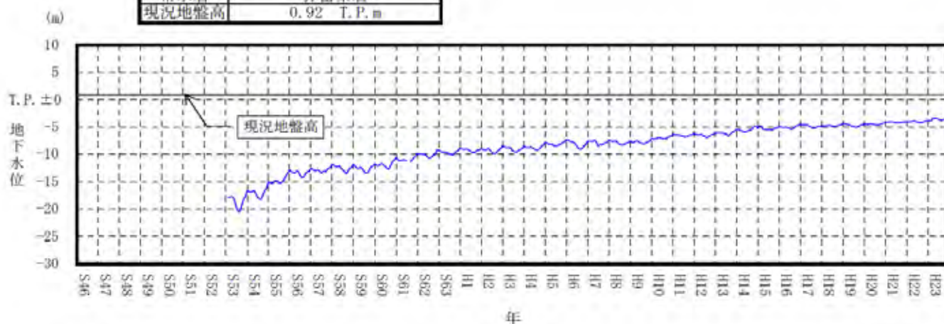
付図-2(17) 地下水位変動図（熱田）
