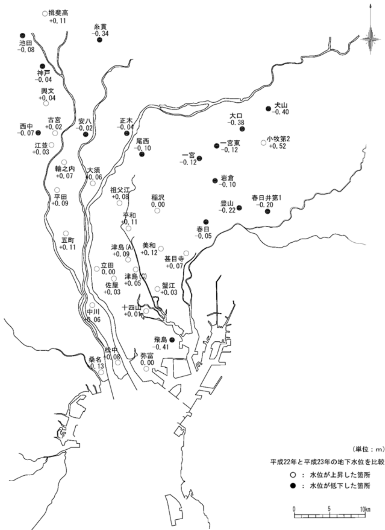
図-11(1) 年平均地下水位の変動量図 [第一礫層(G1)]
