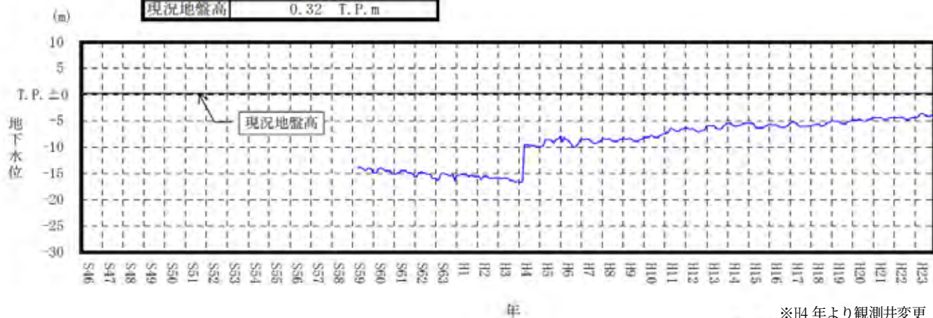
付図-2(14) 地下水位変動図 (千年)
