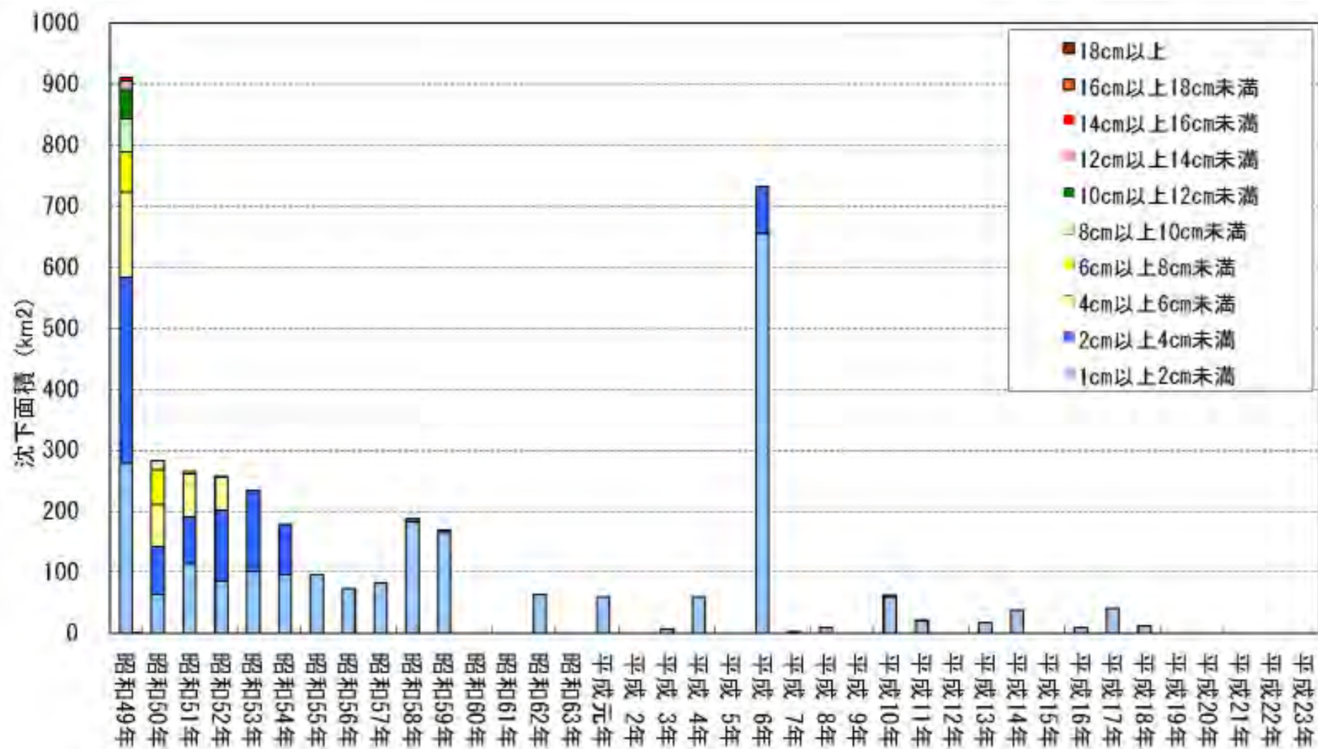
図－2 年間1cm以上の沈下面積
