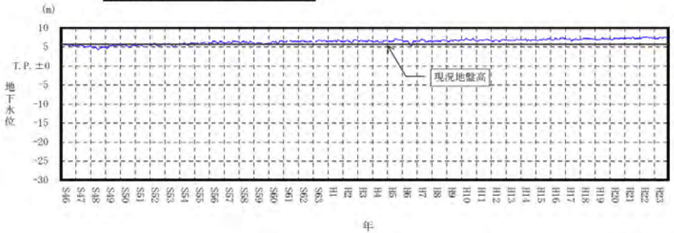
付図-2(11) 地下水位変動図（墨俣）
