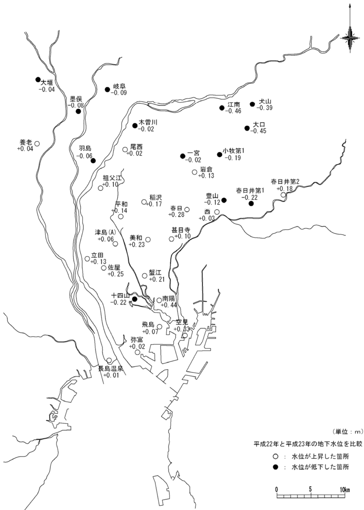
図-11(3) 年平均地下水位の変動量図 [第三礫層(G3)]
