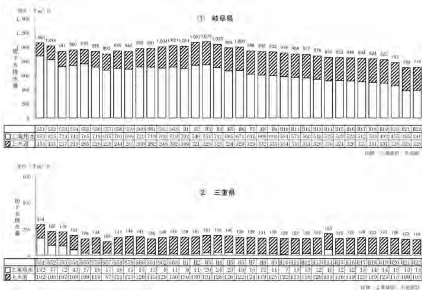
図-18 濃尾平野地盤沈下防止対策要綱の観測地域における地下水揚水量
