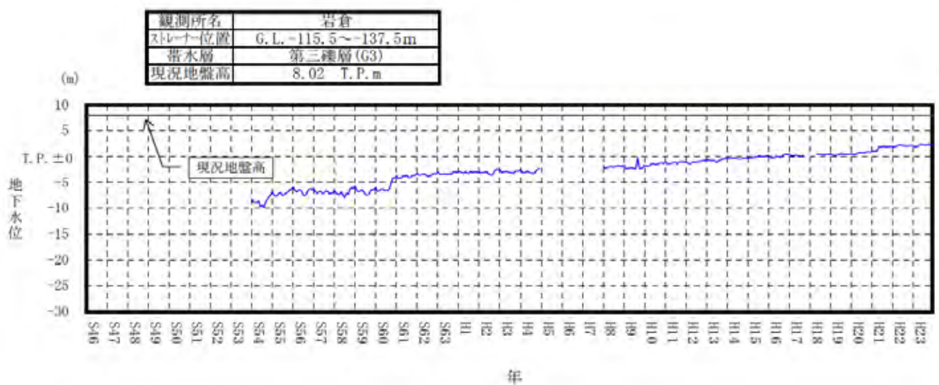
付図-2(21) 地下水位変動図 (岩倉)
