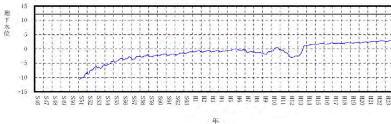
付図-2(7) 地下水位変動図 (安井)
