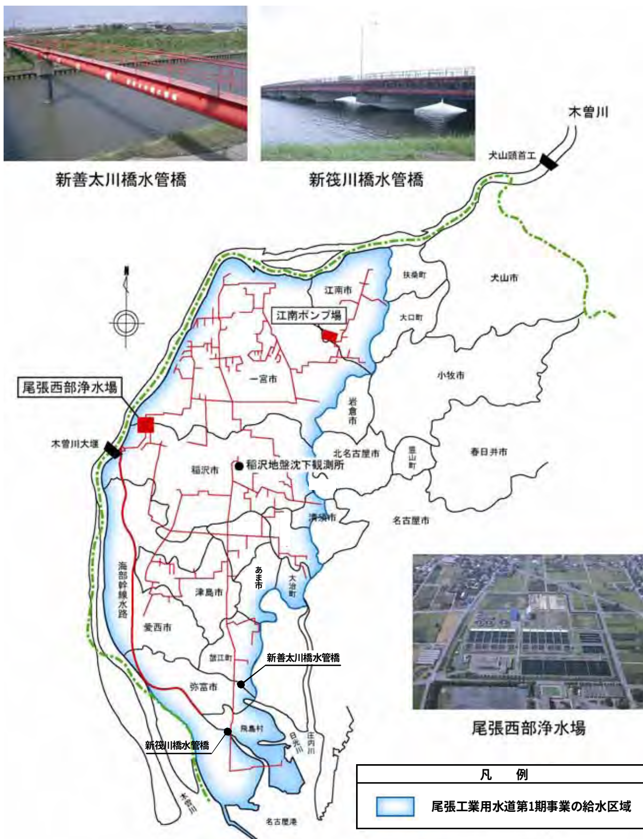
図－13 尾張工業用水道第1期事業の給水区域および稲沢地盤沈下観測所位置図
