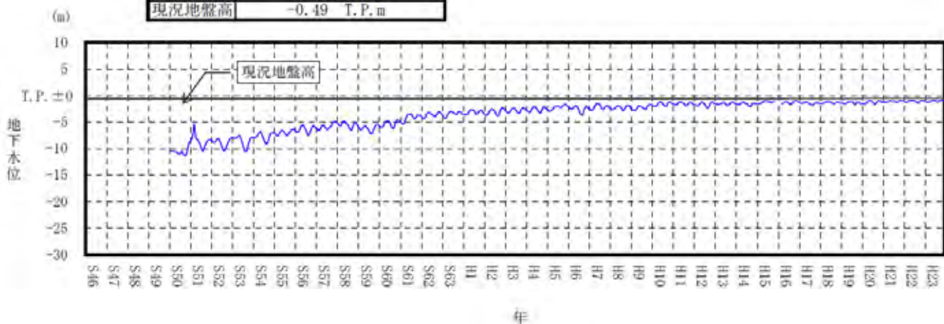
付図-2(19) 地下水位変動図（中川）
