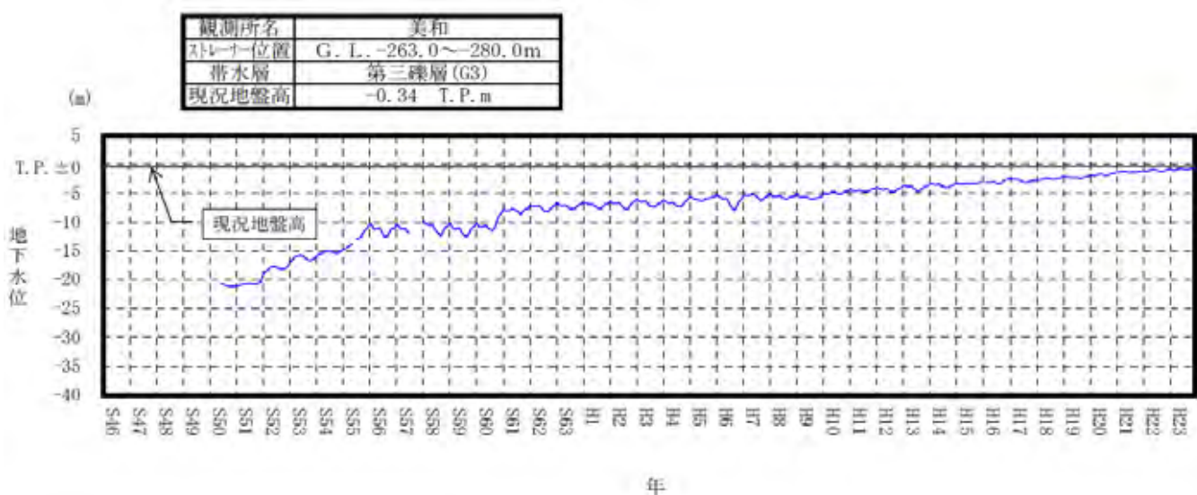
付図-2(6) 地下水位変動図 (美和)
