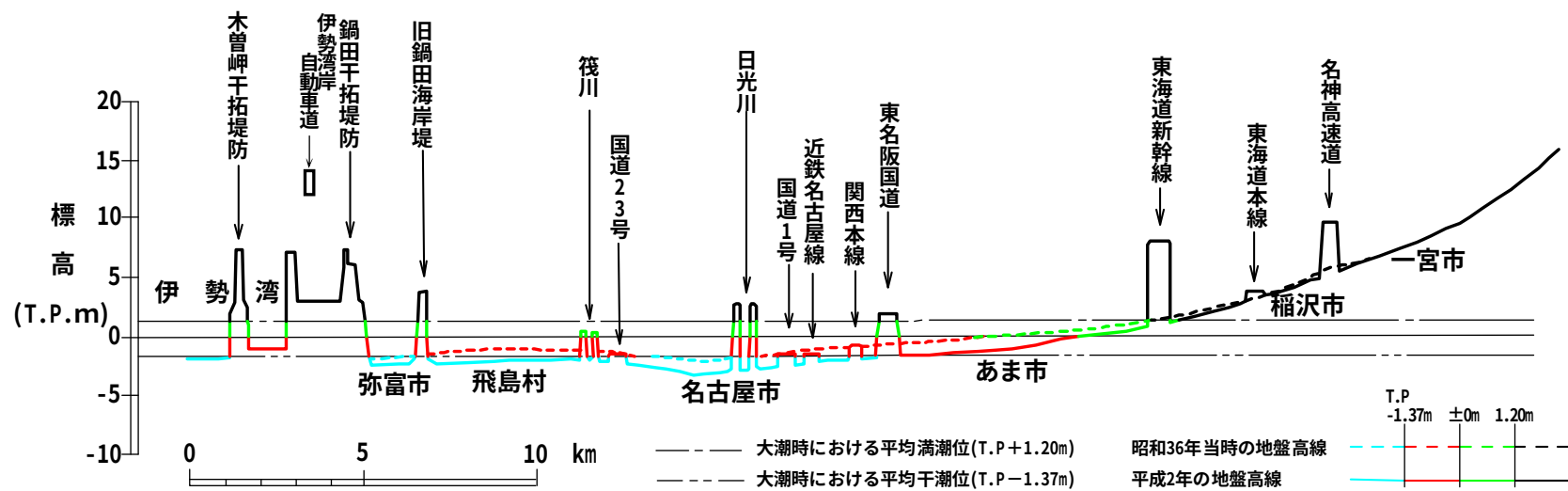
図-10(1) A-A' 断面図
