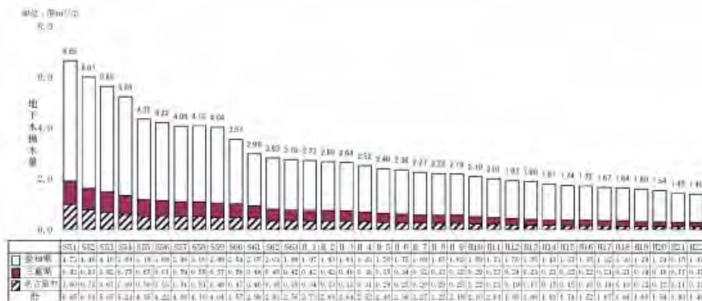
図-17(2) 濃尾平野地盤沈下防止対策要綱の規制地域における地下水揚水量（年間） （工業用水法および環境保全条例による規制地域内）
