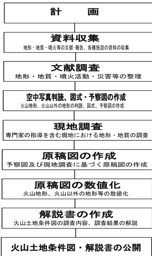
図-3 火山土地条件図の作成フロー
