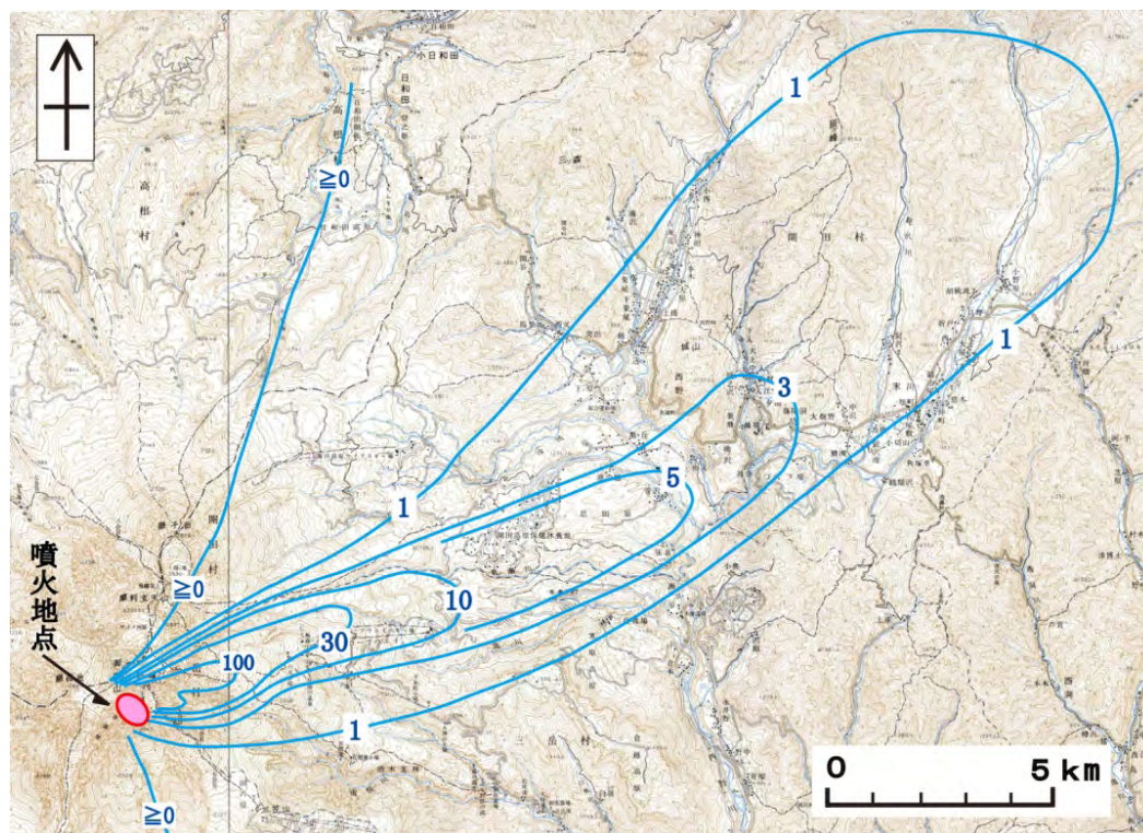
図-12 1979年噴火による火山灰の分布 単位：mm,（小林，1980に基づく）
