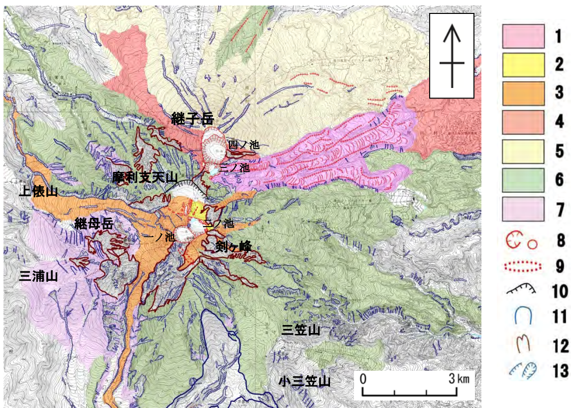
1：三ノ池火山溶岩流 2：二ノ池火山 3：一ノ池火山 4：四ノ池火山 5：継子岳火山 6：摩利支天火山群の前期火山群 7：継母岳火山群 8：火口 9：1979年噴火火口列 10：カルデラ 11：御嶽崩れ 12：大崩壊地 13：崩壊地・崖
