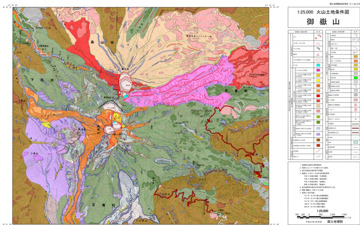
図-1 1:25,000 火山土地条件図「御嶽山」全体図
