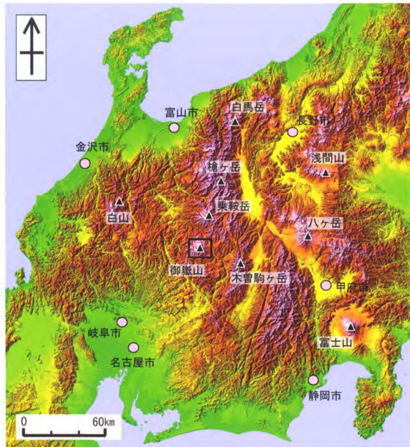
図-4 火山土地条件図「御嶽山」の位置
