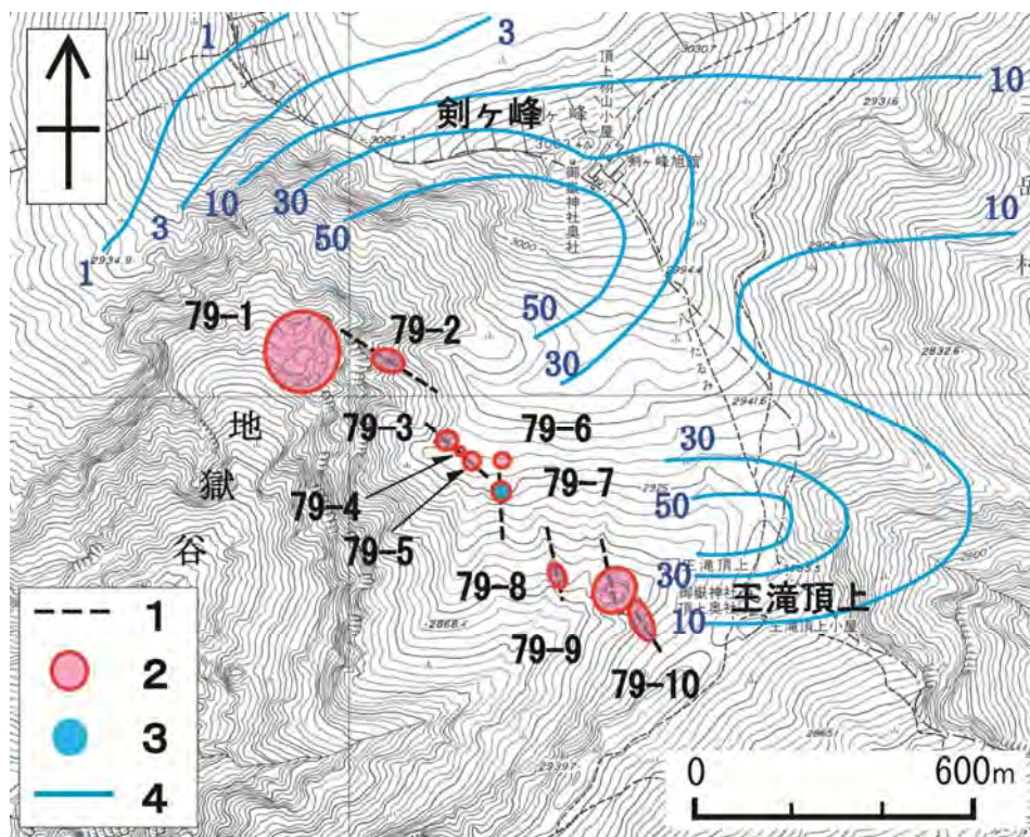
図-11 1979年噴火による火口と降下火山灰の層厚
