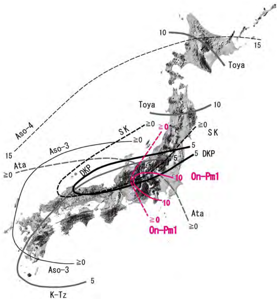
図-9 御岳第1テフラ（On-Pm1）と同時代の広域テフラの分布範囲 降下テフラの厚さ（cm）. 町田・新井（2003）を基に作成
