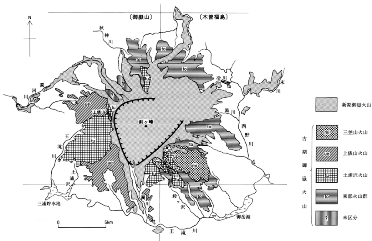
図-8 古期御嶽火山を構成する火山群の分布図 竹内ほか（1998）による
