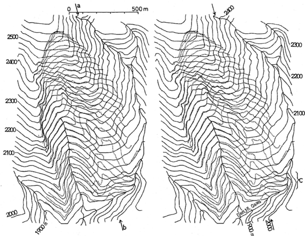
図-14 「御嶽崩れ」前・後の立体地形図（立体視可能）
