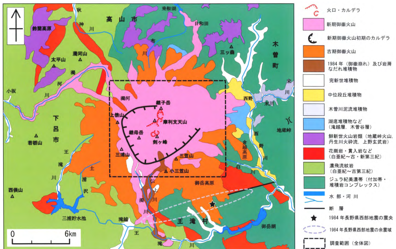
図-5 御嶽火山とその周辺の地質 山田・小林 (1988), 竹内ほか (1998), 新版長野県地質図作成委員会 (2010) を基に作成
