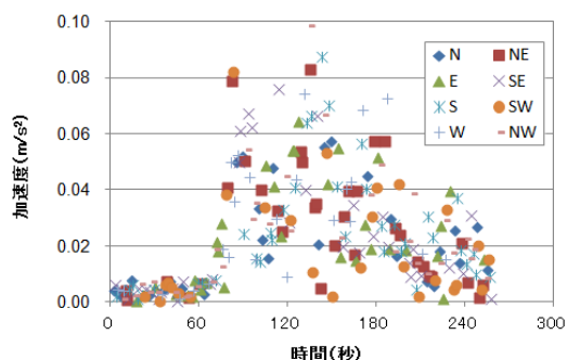
図-12 図-9から計算した8方位別の加速度の時間変化（西向きの 0.39\text{m/s}^2 を省略） 横軸の0は、14時46分0秒である。
