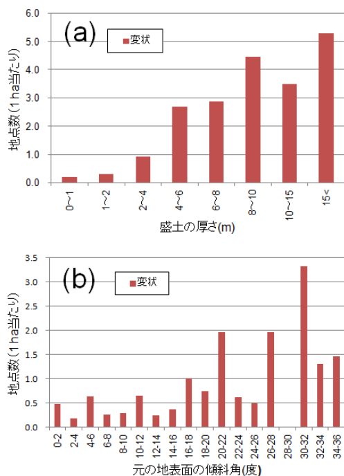
図－7 盛土の厚さと1956年DEMの傾斜角に応じた盛土分布域における変状地点数(1ha当たり地点数；佐藤・中埜, 2011を修正)
