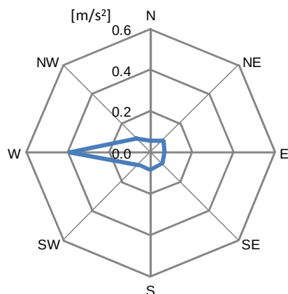
図-11 図-9から計算した方位別最大加速度
