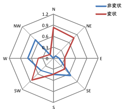
図－8 2000年DEMの斜面方位に応じた盛土分布域における変状・非変状地点数(1ha当たり地点数；佐藤・中埜, 2011を修正)
