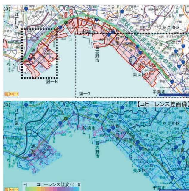
図－7 (a)東京湾岸沿いの液状化発生領域。国土交通省関東地方整備局・地盤工学会（2011）をもとに作成。赤色及び青色の部分はそれぞれ液状化範囲、非液状化範囲を示す。(b)2011/1/4-2011/2/19のコヒーレンス画像と2011/2/19-2011/4/6のコヒーレンス画像の差画像。コヒーレンスが低下したことを示す紫～黄色が部分的に見られる。
