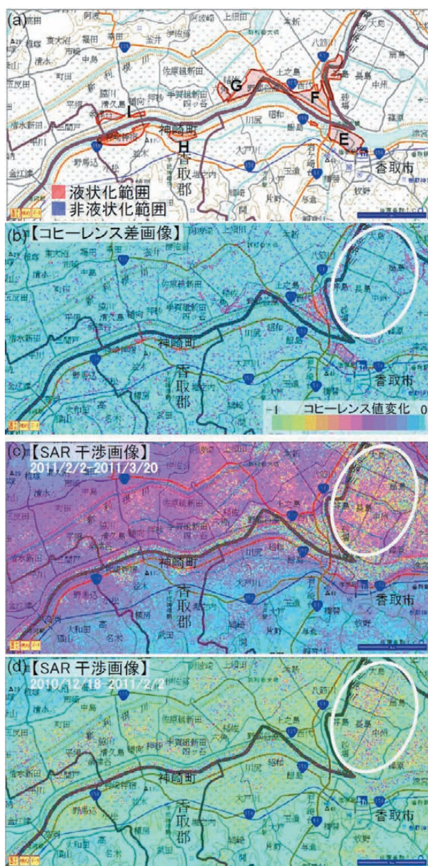
図－6 (a)香取市・稲敷市及びその周辺の液状化発生領域、(b)コヒーレンス差画像、(c) (d) SAR干渉画像。コヒーレンス差画像は図－2 (b)と同じである。SAR干渉画像(c)及び(d)はそれぞれ2011/2/2-2011/3/20及び2010/12/18-2011/2/2のデータペアによる解析結果。
