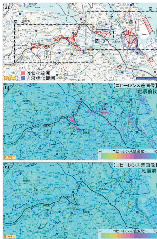
図-2 (a)利根川下流域の液状化発生領域。国土交通省関東地方整備局・地盤工学会(2011)をもとに作成。赤色及び青色のマスク領域はそれぞれ液状化範囲、非液状化範囲を示す。
