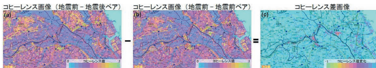
図-1 コヒーレンス差画像の作成. (a)地震前-地震後データペアによる干渉処理から得られたコヒーレンス画像. (b)地震前-地震前データペアによる干渉処理から得られたコヒーレンス画像. (c) コヒーレンス画像(a)のコヒーレンス値からコヒーレンス画像(b)のコヒーレンス値を差し引いて作成したコヒーレンス差画像.
