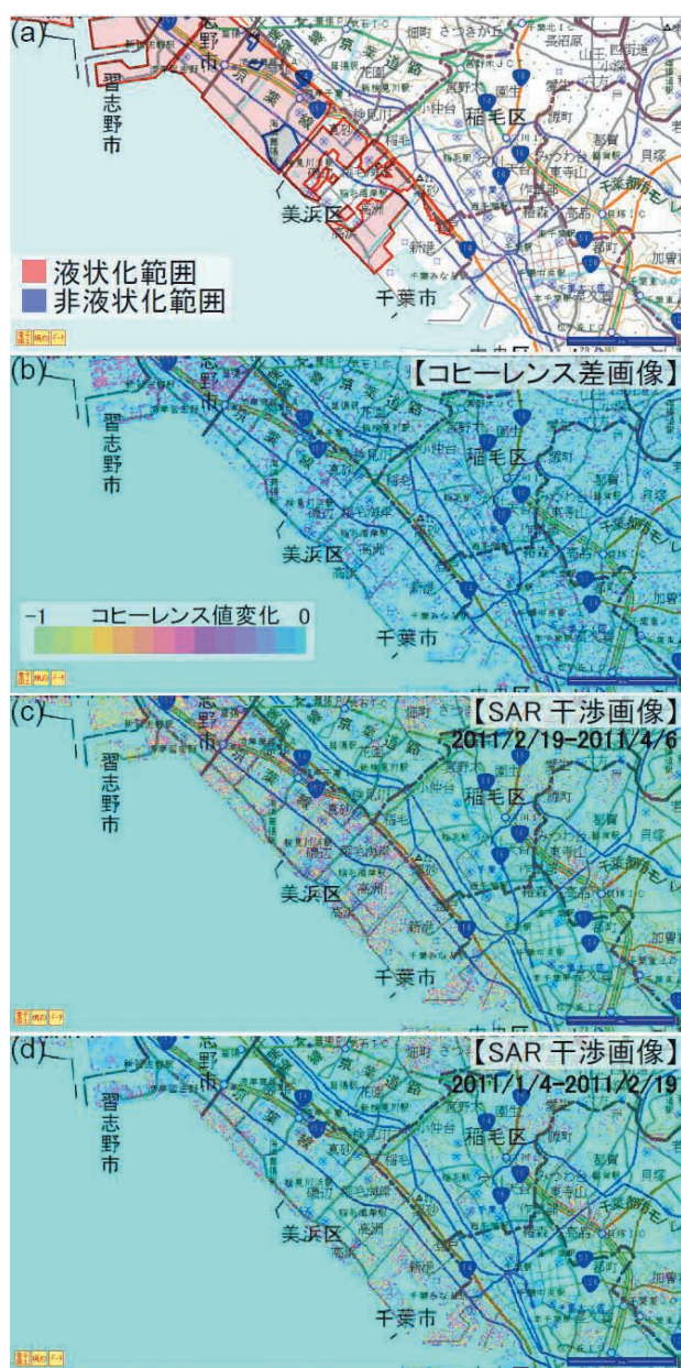
図ー10 習志野市～千葉市の湾岸沿いの液状化発生領域 (a), コヒーレンス差画像 (b), SAR 干渉画像 (c) (d). コヒーレンス差画像は図ー7 (b) と同じ. SAR 干渉画像はそれぞれ 2011/2/19-2011/4/6 及び 2011/1/4-2011/2/19 のデータペアによる解析結果.
