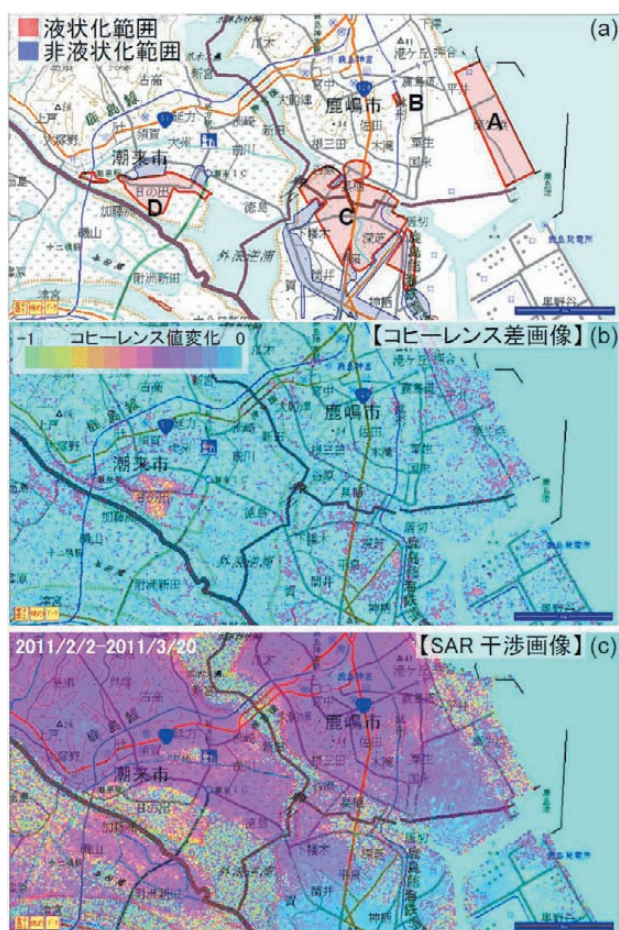
図－3 (a)潮来市・鹿嶋市及びその周辺の液状化発生領域，(b)コヒーレンス差画像，(c)SAR干渉画像．コヒーレンス差画像は図－2 (b)と同じである．SAR干渉画像は2011/2/2-2011/3/20のデータペアによる解析結果．
