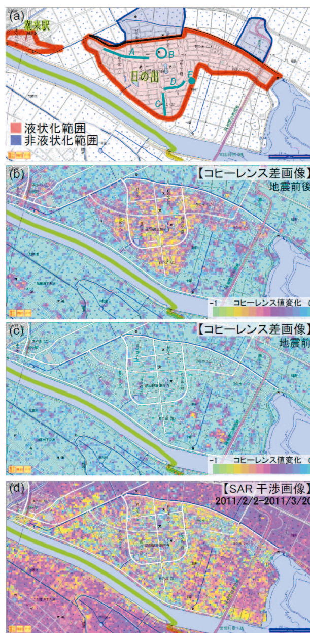
図－4 (a)潮来市日の出地区及びその周辺の液状化発生領域，(b) (c)コヒーレンス差画像，(d)SAR干渉画像．図－4 (a)のA～Eは，図－5に示す写真の撮影場所を示す．コヒーレンス差画像(b)及び(c)はそれぞれ図－2 (b)及び(c)と同じである．SAR干渉画像は2011/2/2-2011/3/20のデータペアによる解析結果．
