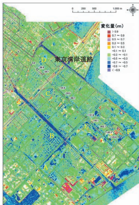
図-26 航空レーザ測量による標高差分図と水準測量による相対沈下量の重ね合わせ
