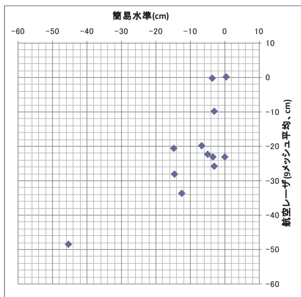
図-27 水準測量による街区基準点の沈下量と航空レーザ差分図による変化量との関連性
