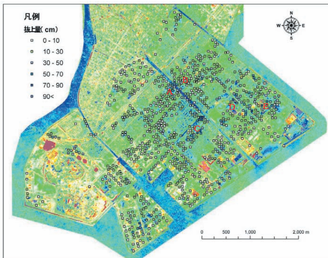
図-28 杭基礎建物の抜け上がり量（千葉県環境研究センター，2011b）と航空レーザ測量による標高差分図との重ね合わせ（航空レーザ差分図の凡例は図-26 と同じ．抜け上がり量の色は航空レーザ差分図の色と同様）
