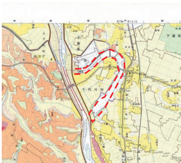
図-16 下妻市鬼怒周辺の土地条件図 破線は旧河道
