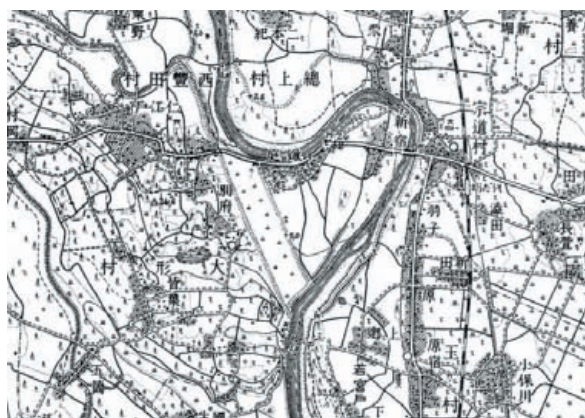
図-18 昭和 9 年修正 5 万分 1 地形図「水海道」
