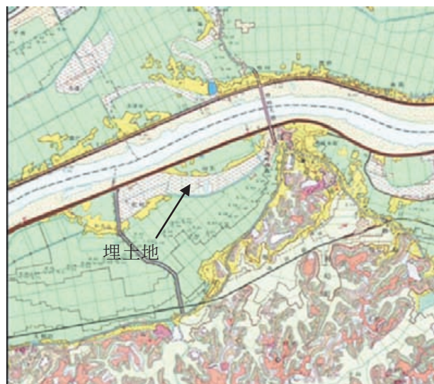
図－8 千葉県神崎町付近の土地条件図 （土地条件図「佐原」の一部）
