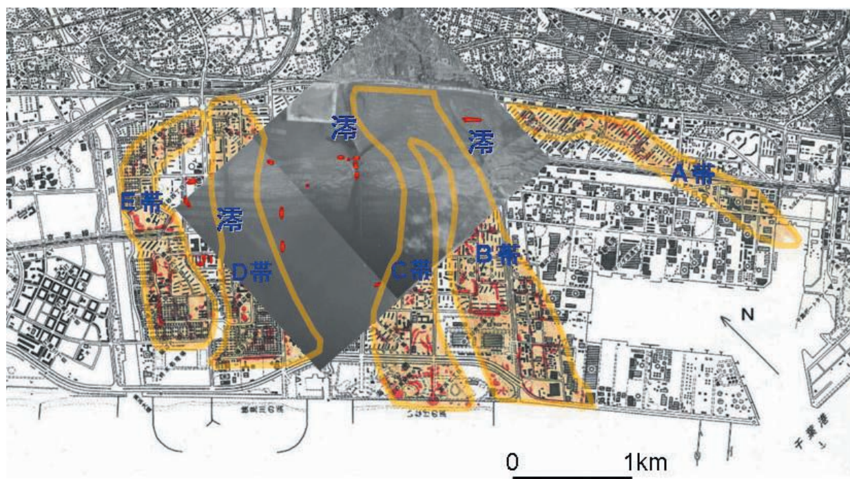
図-24 千葉市美浜区における噴砂の分布と埋め立て前の空中写真(MKT61-3 C6-1~2)との重ね合わせ 噴砂の分布は千葉県環境研究センター(2011a)による
