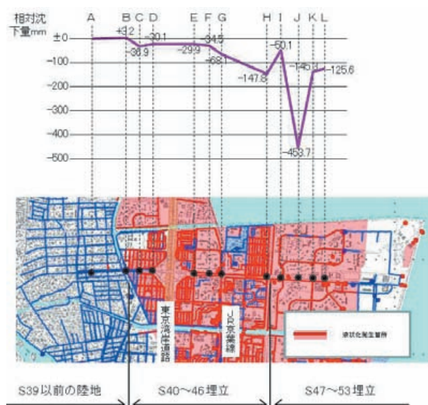
図-25 浦安市における沈下量の測量結果
