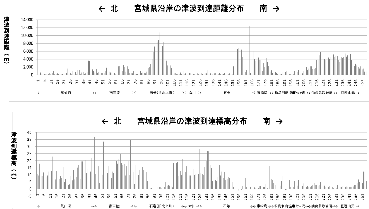
図－3 津波到達距離と到達標高
