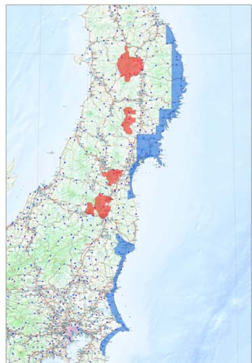
図-9 高精度標高データ整備地域図
