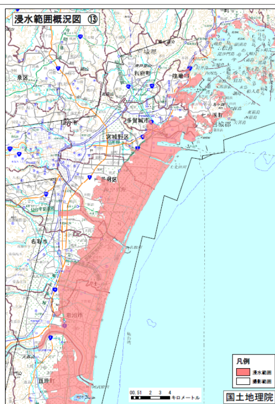
図-2 浸水範囲概況図出力例
