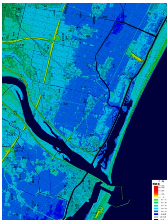
図－10 デジタル標高地形図（名取川河口付近：震災前） 図－11 デジタル標高地形図（名取川河口付近：震災後）
