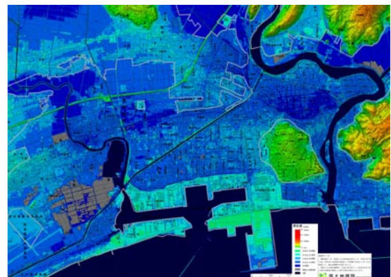
図－4 デジタル標高地形図 (石巻付近)
