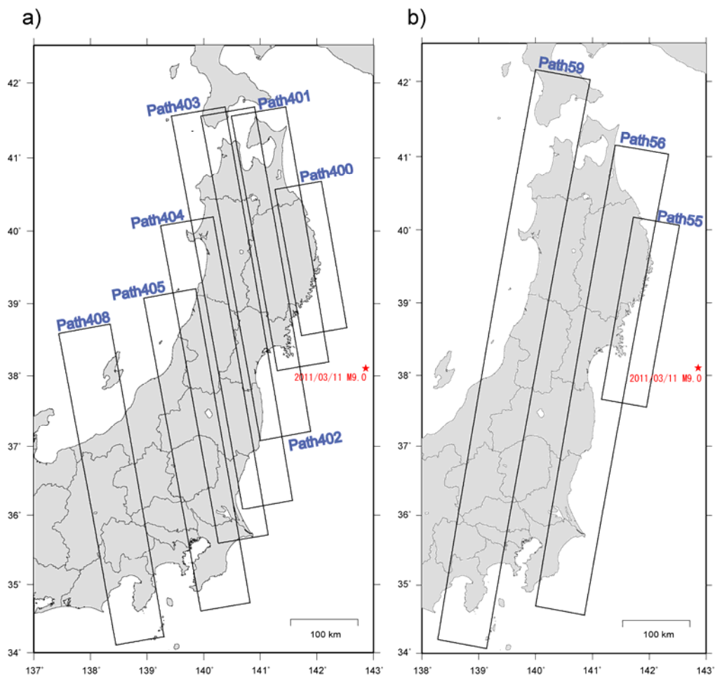
図－１ 緊急解析の範囲 a) 北行軌道 b) 南行軌道
