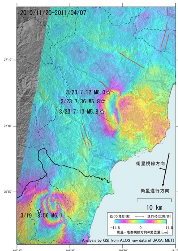
図-6 SAR干渉解析図(茨城県北部の地震(3/19)及び福島県浜通りの地震(3/23))
