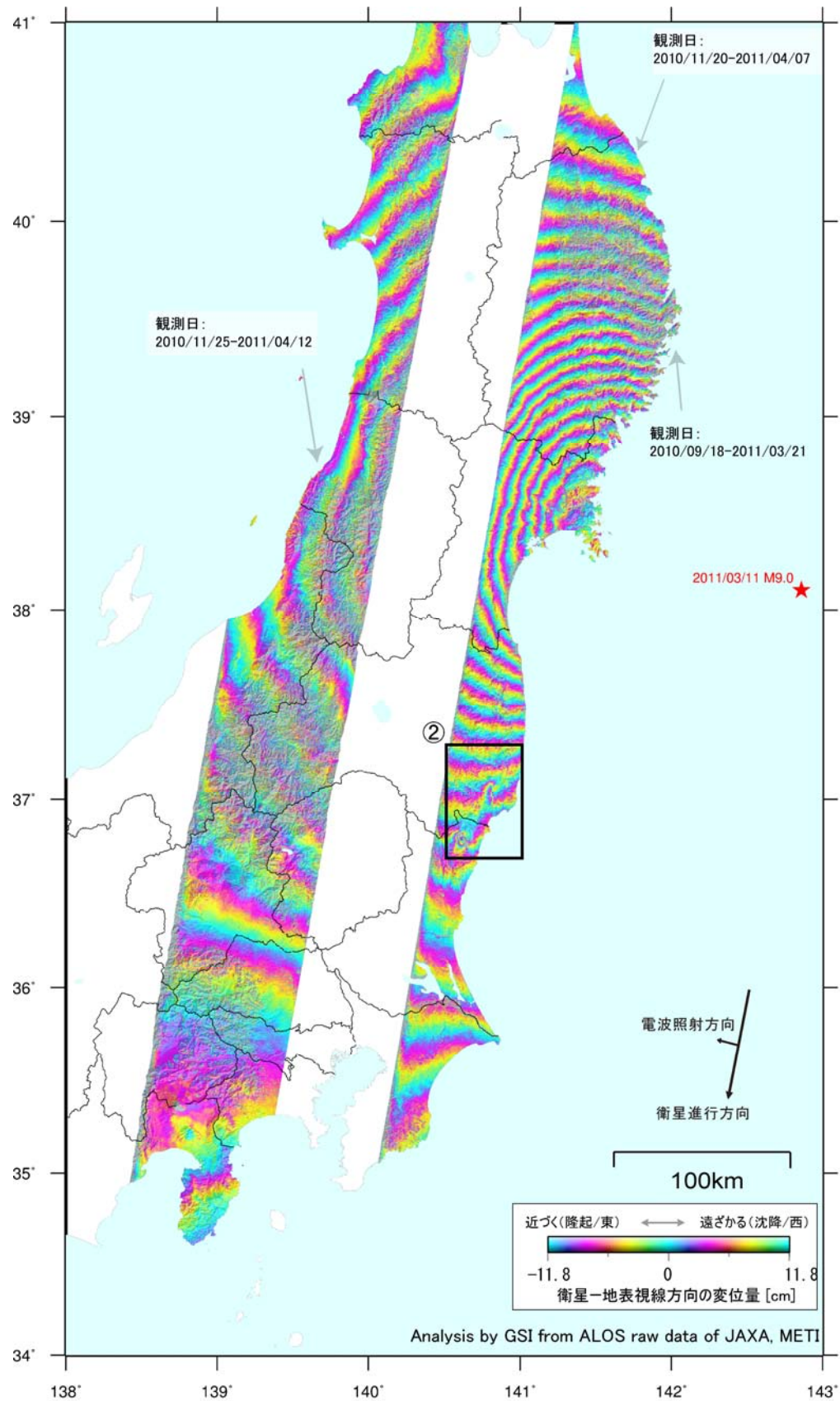
図ー3 南行軌道による SAR 干渉解析画像図
