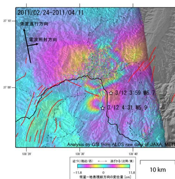
図-5 SAR干渉解析図(長野県・新潟県県境付近の地震(3/12))
