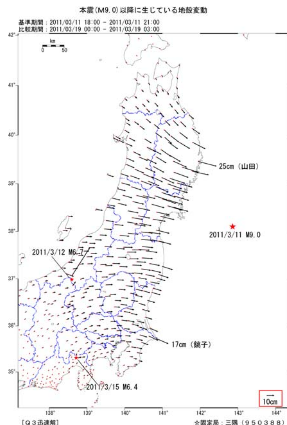
図ー1 地震後の水平地殻変動（3月11日ー3月19日：Q3解）
