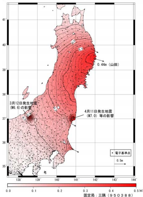
図－2 地震後の地殻変動等変動量線図(3月11日－4月17日:Q3解及びR3解)(a) 水平変動量 (b) 上下変動量
