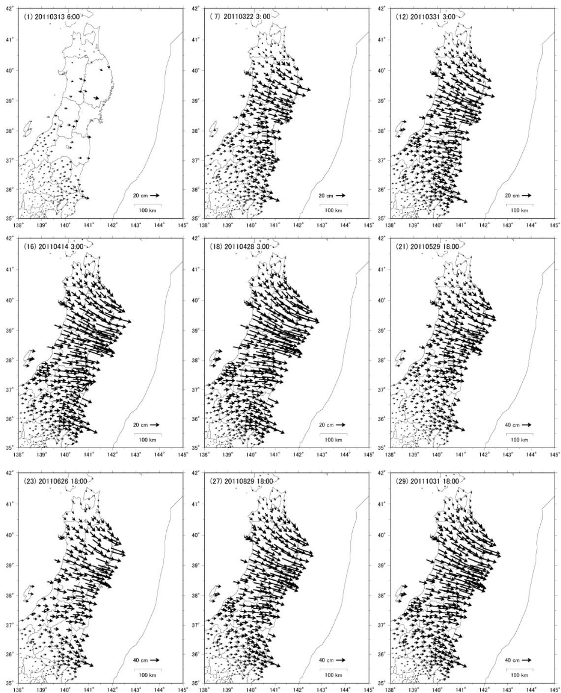
図－4 地震後の地殻変動（水平変動）
