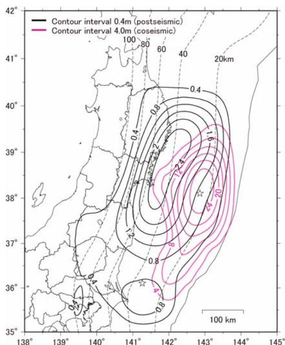
図－7 地震時と余効すべり分布の比較
