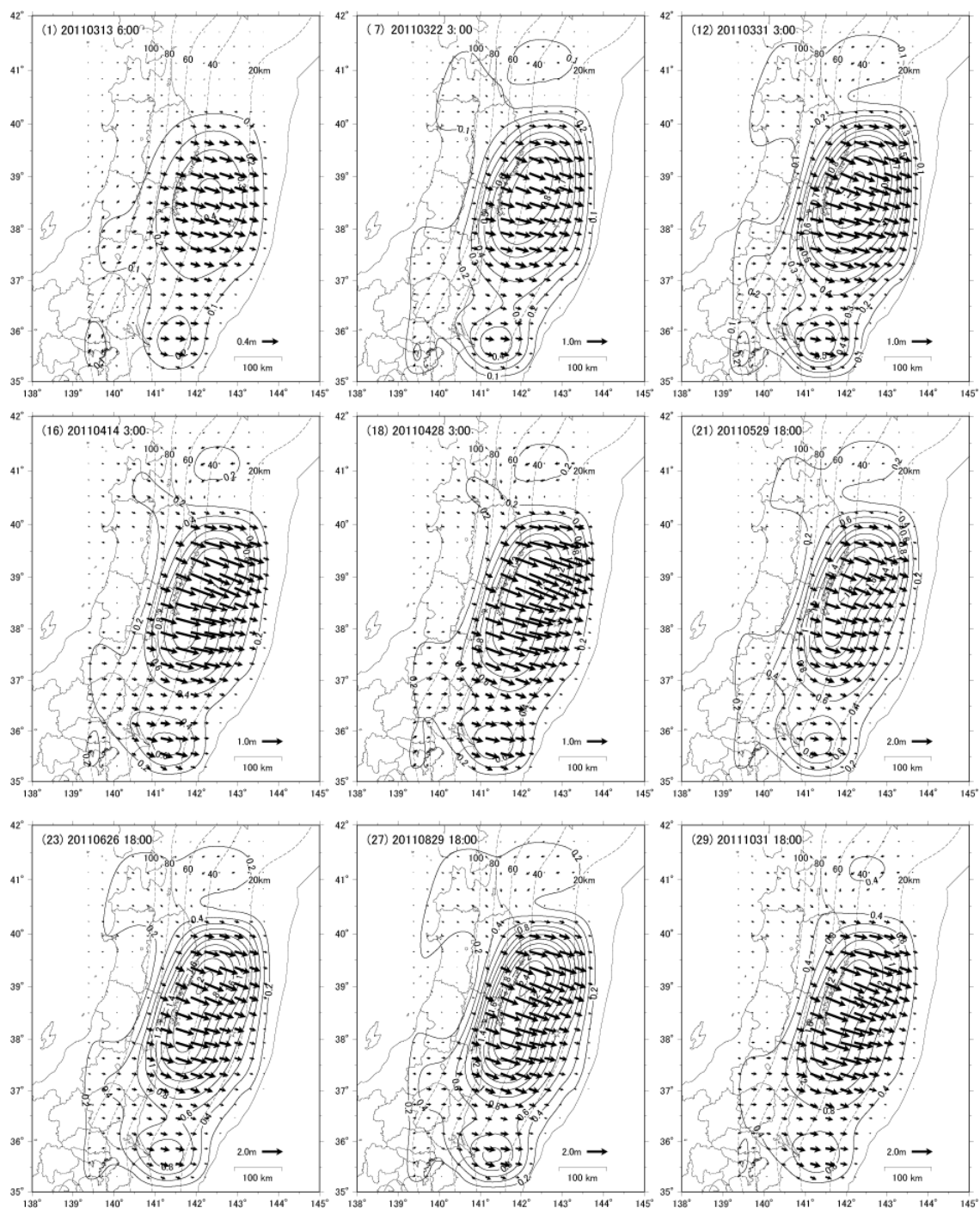
図-6 余効すべり分布
