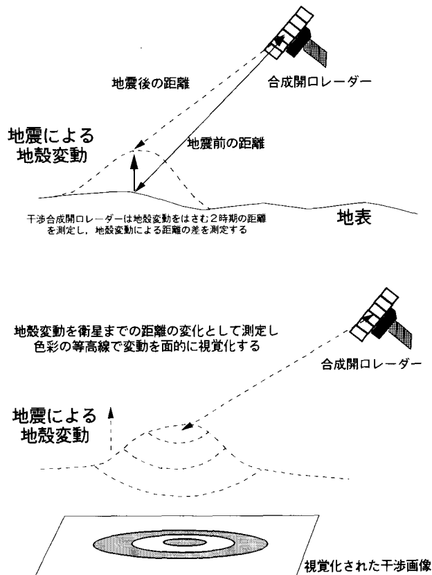
図-2 干渉SARの原理図
