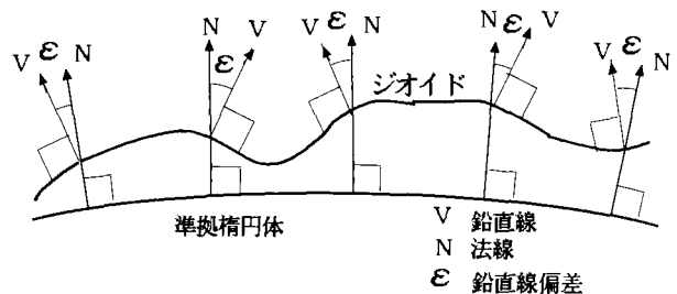
図3 鉛直線偏差
