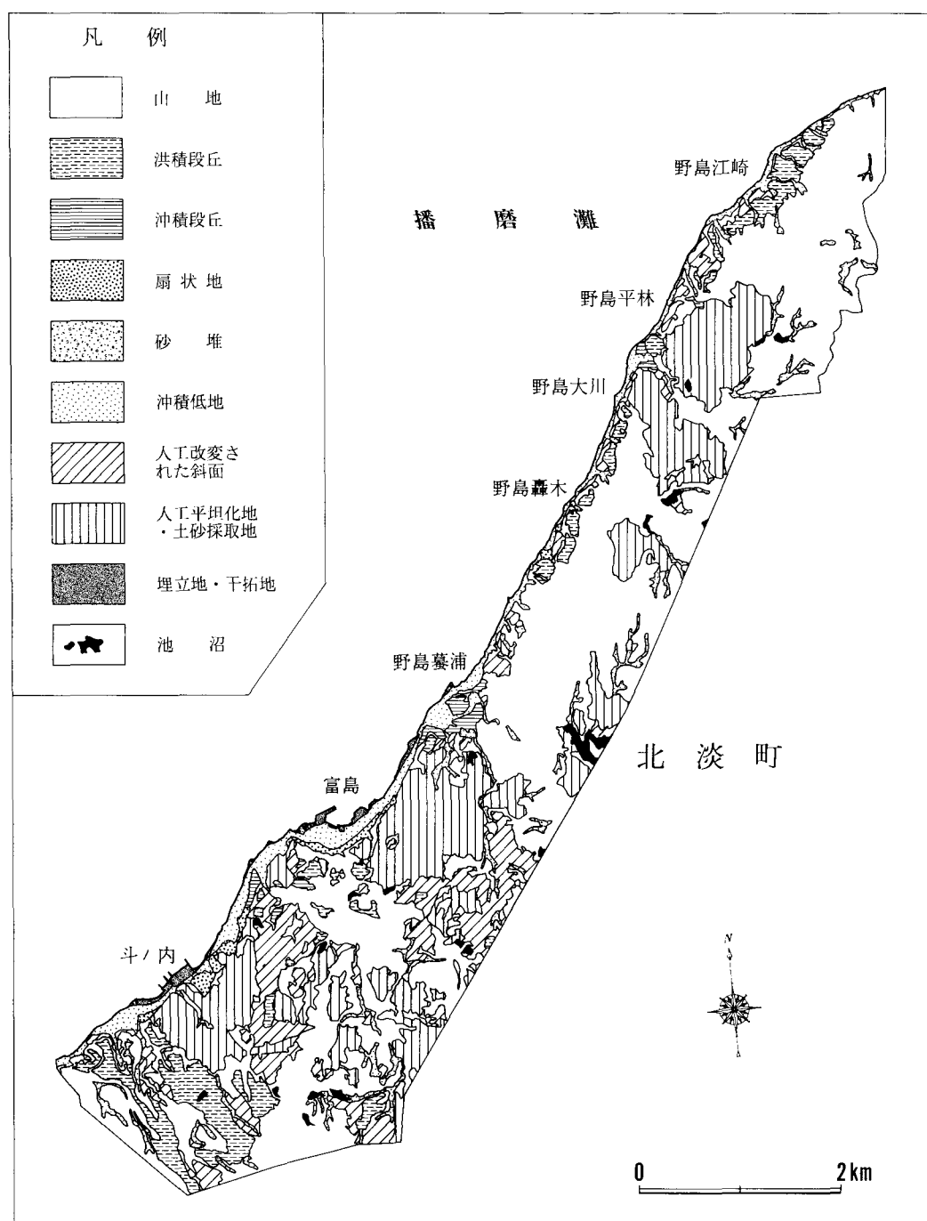
図-4 変位量計測地域の地形分類図
