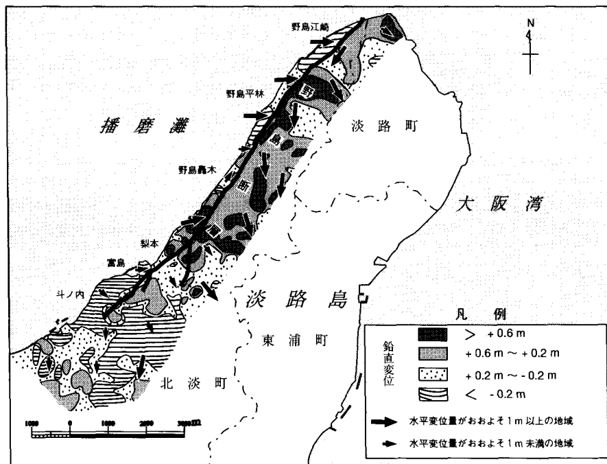
図-3 水平および鉛直変位分布の概要 地震断層のトレースは栗田ほか(1996)による。
