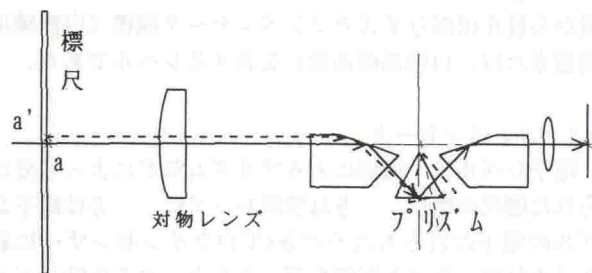
図-6 ヒステリシス誤差
