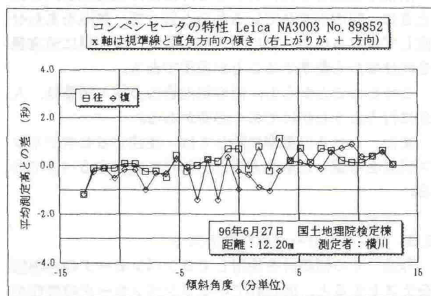
図-5 コンペンセータの特性
