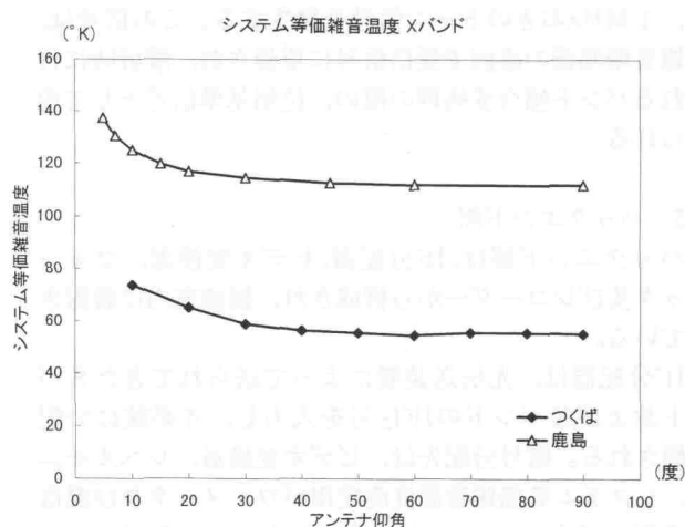
図-2 システム等価雑音温度
