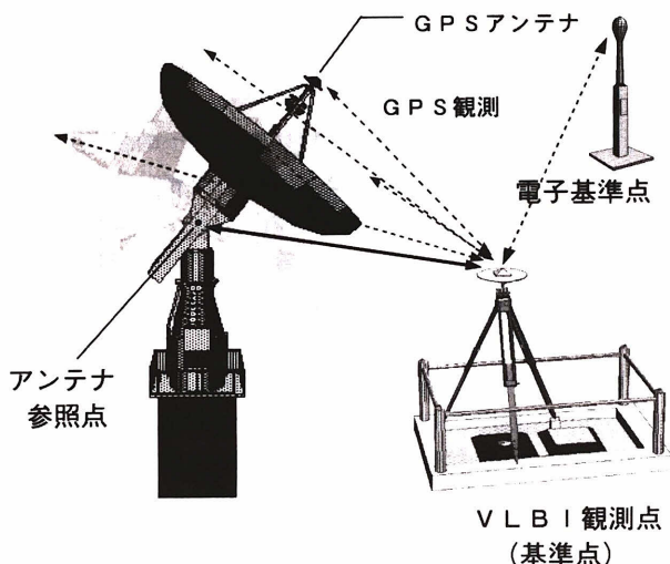
図-1 GPSを用いた取り付け測量
