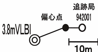
図－7 新十津川における基準点の位置関係
