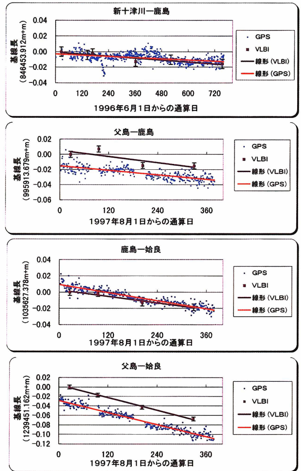
図ー 10 VLBI と GPS の基線長比較
