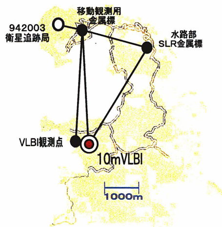
図-5 父島における基準点の位置関係
