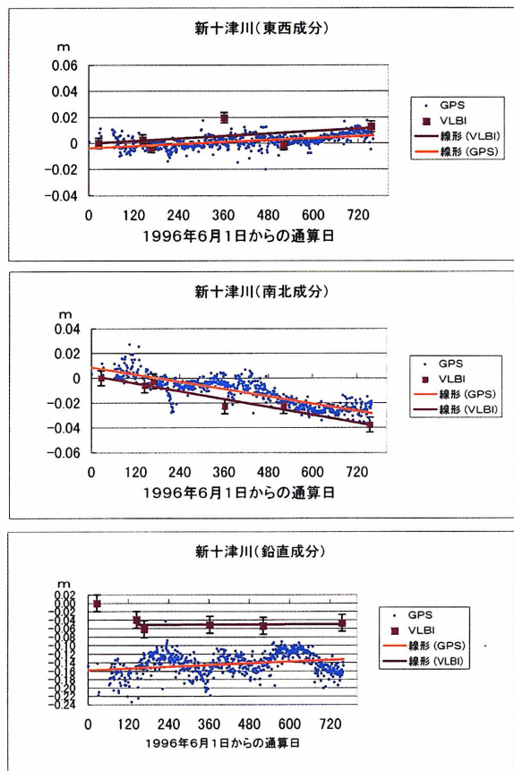
図－11 新十津川局におけるVLBIとGPSの座標比較
