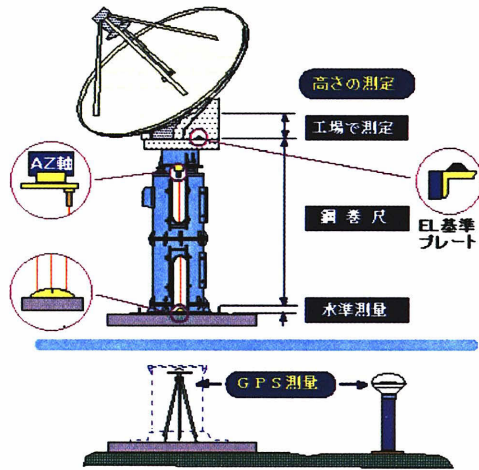
図－3 3.8mVLBIアンテナ取り付け測量
