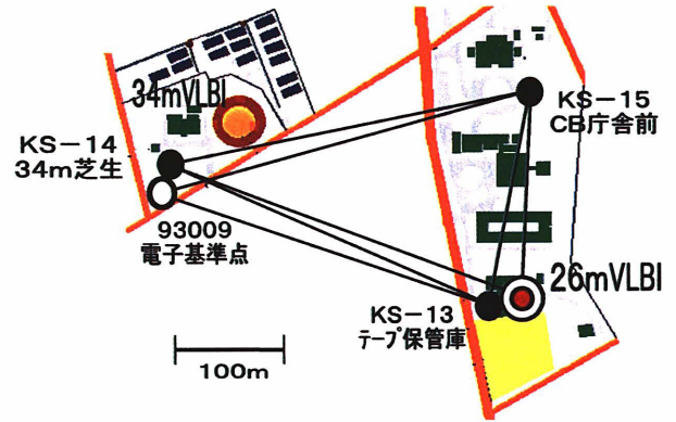
図－4 鹿島における基準点の位置関係
