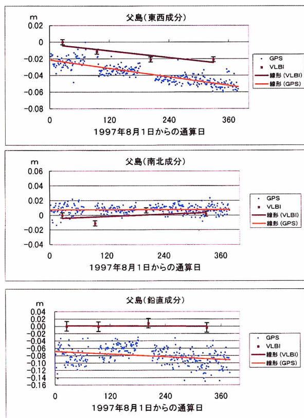
図-13 父島におけるVLBIとGPSの座標比較
