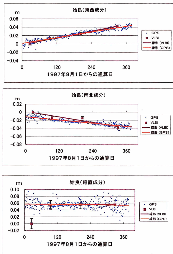
図－12 始良におけるVLBIとGPSの座標比較
