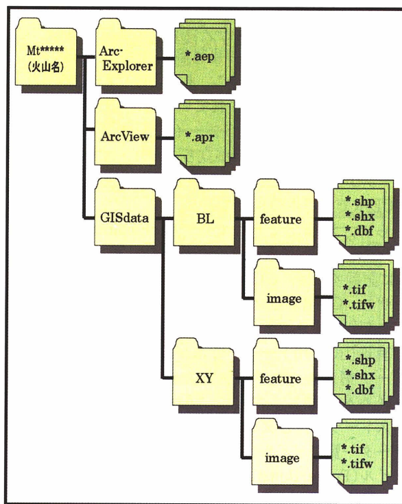
図-1 火山災害対策GIS用データの構造
