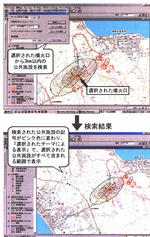
図－7 2つの情報の相互関係による検索・選択表示例
