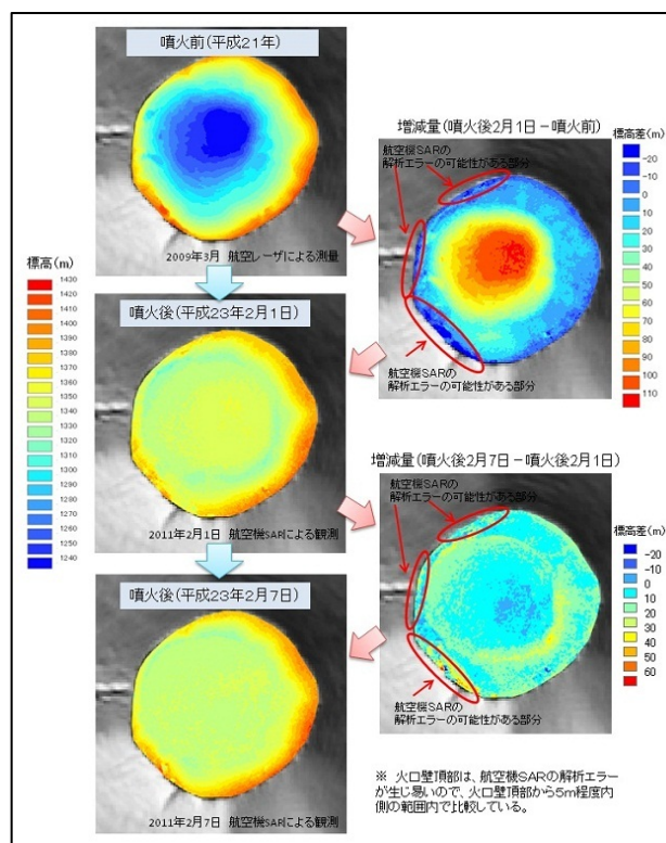
図-8 噴火前後の火口内の標高値変化
