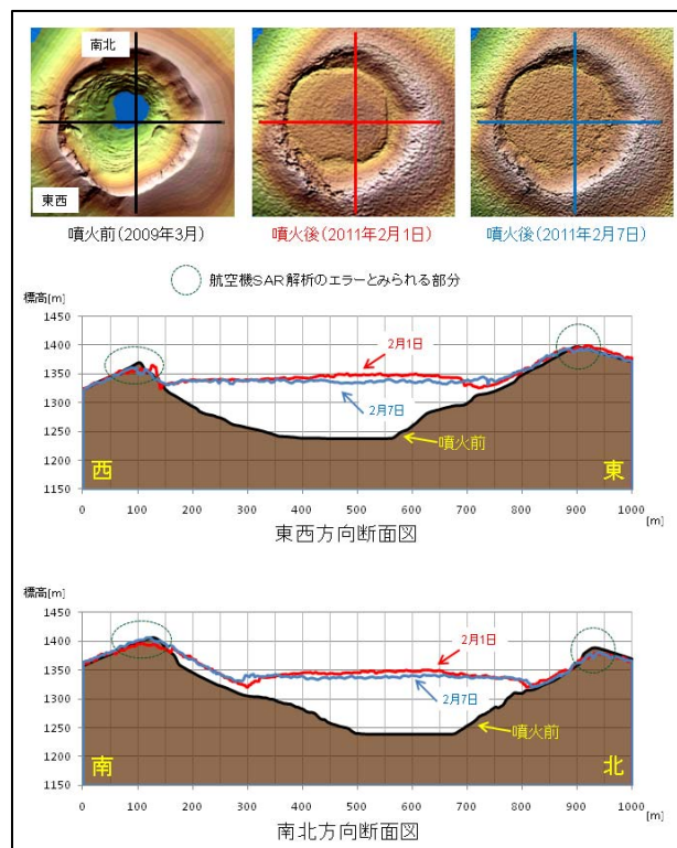
図-9 噴火前後の火口付近断面図
