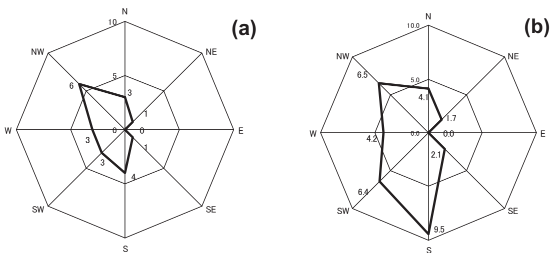
図-5 北海岸における斜面崩壊と斜面方位の関係。(a) 斜面崩壊の斜面方位に関する頻度、(b) 各斜面方位に占める斜面崩壊の比(×1/10,000)
