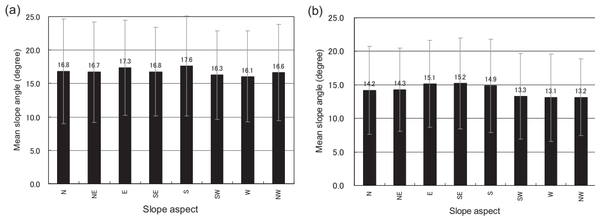
図－7 斜面方位ごとの平均傾斜。エラーバーは標準偏差。(a) は北海岸, (b) は西海岸。
