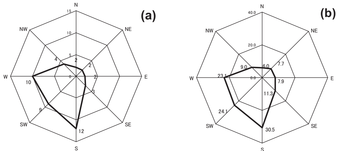
図－6 西海岸における斜面崩壊と斜面方位の関係。(a) 斜面崩壊の斜面方位に関する頻度, (b) 各斜面方位に占める斜面崩壊の比 ( \times 1/10,000 )
