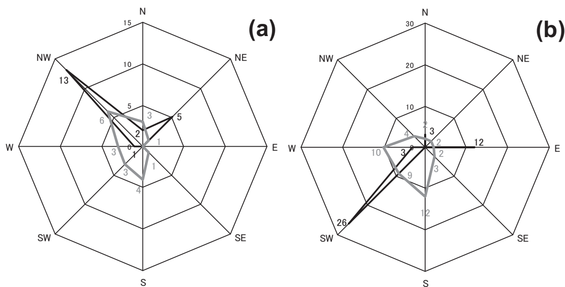
図ー11 崩壊の斜面方位（灰色線）と断層モデルから計算された斜面崩壊箇所における地表変位の方向（黒線）。 断層モデルは小沢ほか（2007）による。（a）北海岸（21ヶ所），（b）西海岸（44ヶ所）
