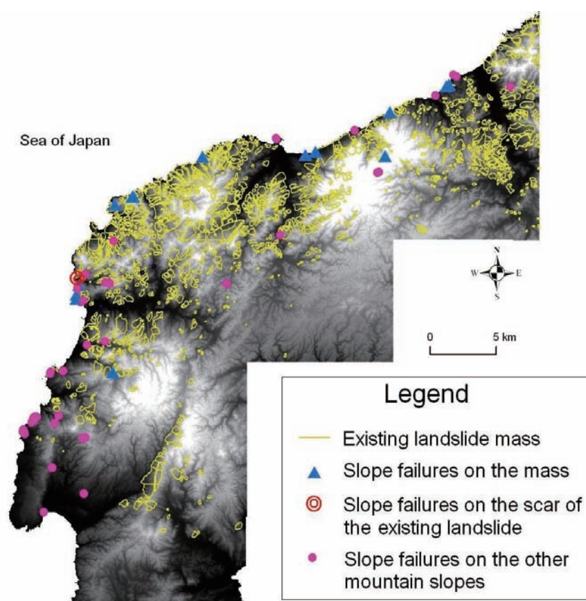
図ー8 斜面崩壊と地すべり地形分布図データベース（防災科学技術研究所，2007）の重ね合わせ。斜面崩壊の位置を既往地すべり地形に応じて3つに分類（青三角：地すべり移動体上で生じた斜面崩壊；赤二重丸：滑落崖上で生じた斜面崩壊；桃色の点：その他の山地斜面で生じた斜面崩壊）した。
