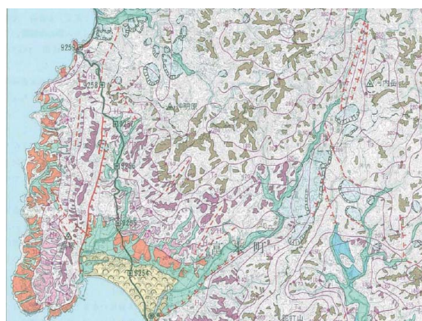
図-3 1/10 万地殻変動土地条件図「能登半島」の一部 (志賀町富来付近, 赤の実線は, 活断層)
