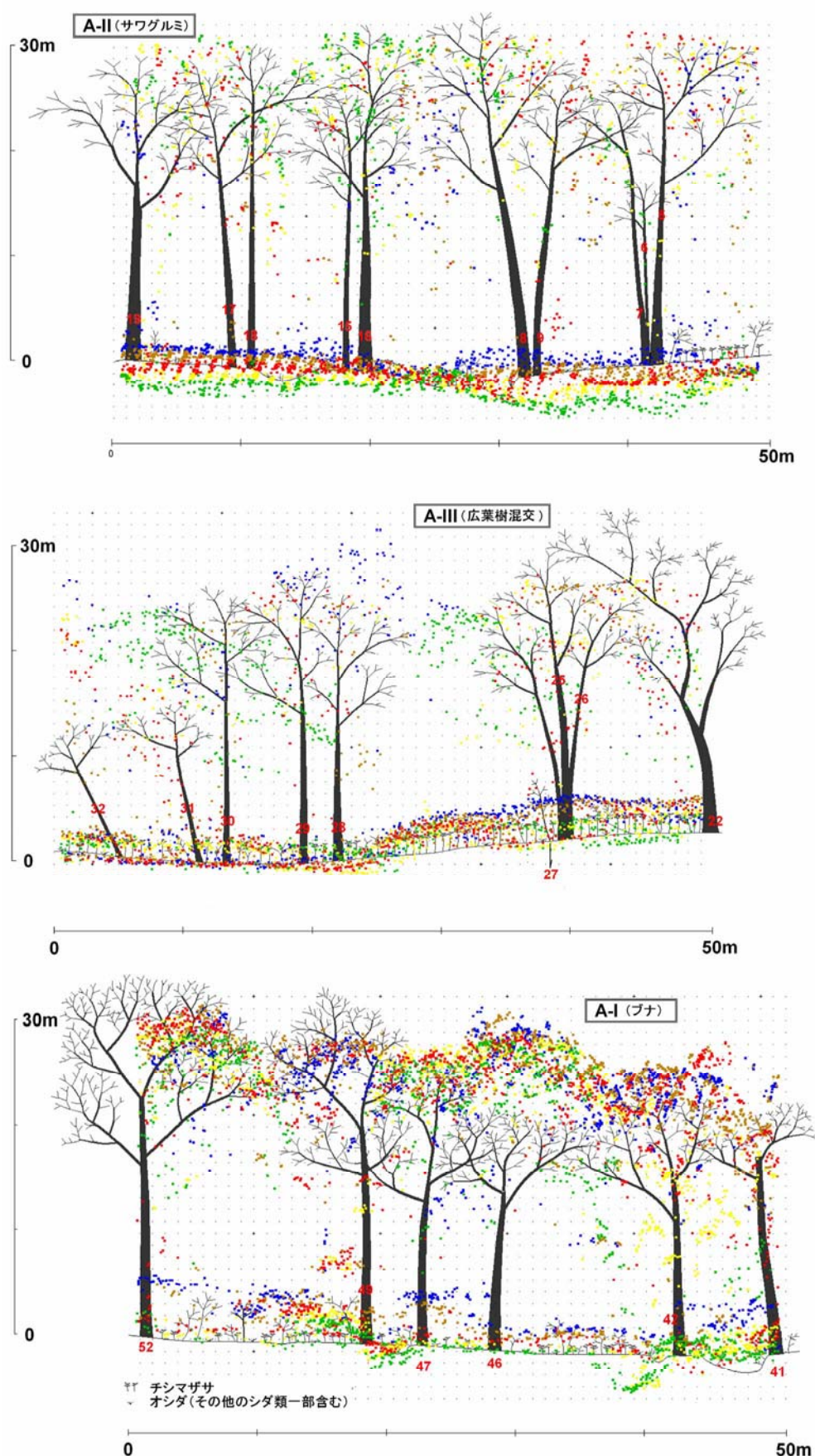
図ー6 植生断面図とレーザ反射点群の重ね合わせ(落葉期)。赤字は、表ー3に示した樹木番号。
