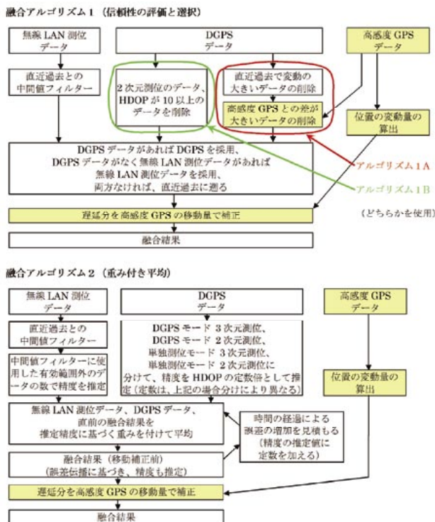
図－3 無線 LAN 測位と GPS を組み合わせた屋内外のシームレス測位のアルゴリズム
