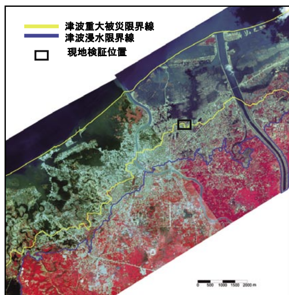
図－5 「津波重大被災限界線」と「津波浸水限界線」
