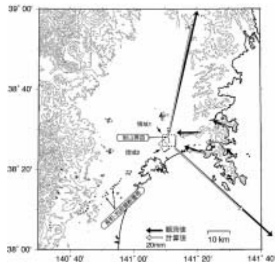
図－2 GPS連続観測点と機動観測点における地震時地殻変動の観測値と計算値。
