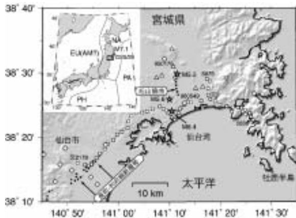
図－1 地殻変動の観測点と地震の震央を示した地形陰影図
