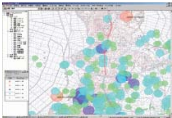
図-6 地震の規模により分類表示(背景: 1/25,000)
