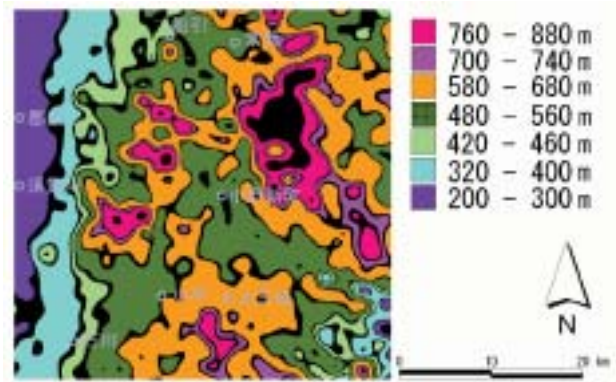
図-9 磐城石川～郡山間の標高帯の平面的分布。
