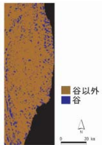
図-11 自動抽出による谷の分布。
