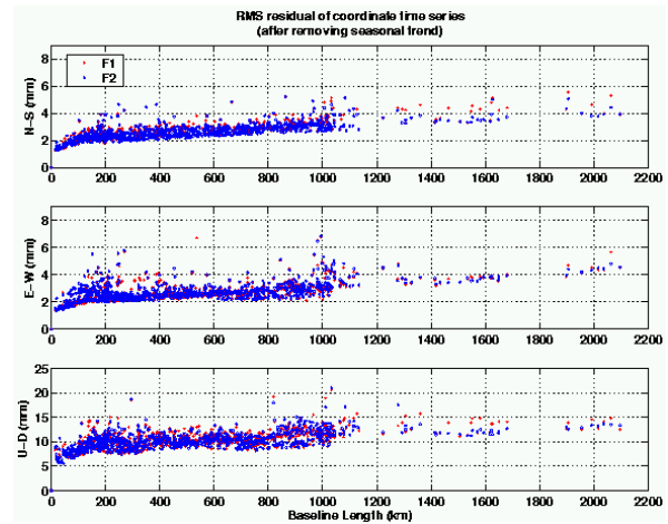
図 1 F1 解及び F2 解の長期再現性の比較
