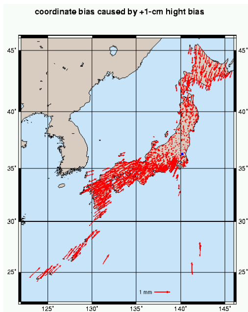
図-6 固定点の高さのバイアスによる間接効果 固定点の a priori 座標の高さ成分を 10mm 上方に変更した場合の、水平座標解の変化。
