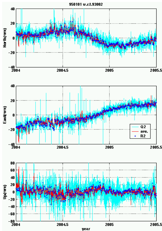
図-3 Q2 解の移動平均の時系列
