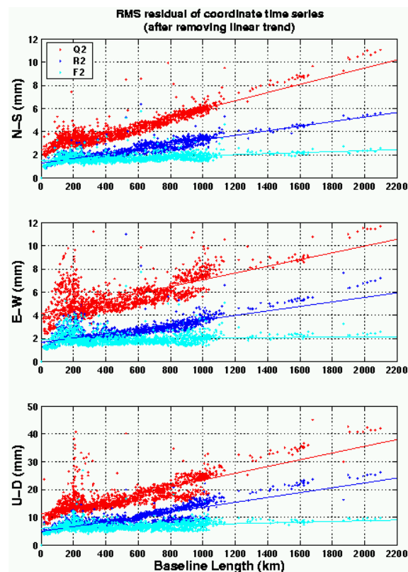
図－2 ルーチン解の短期再現性
